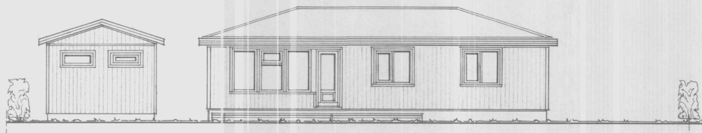
SUÐ - VESTURHLIÐ. 1:100
