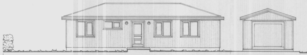
NORÐ - AUSTURHLIÐ. 1:100
