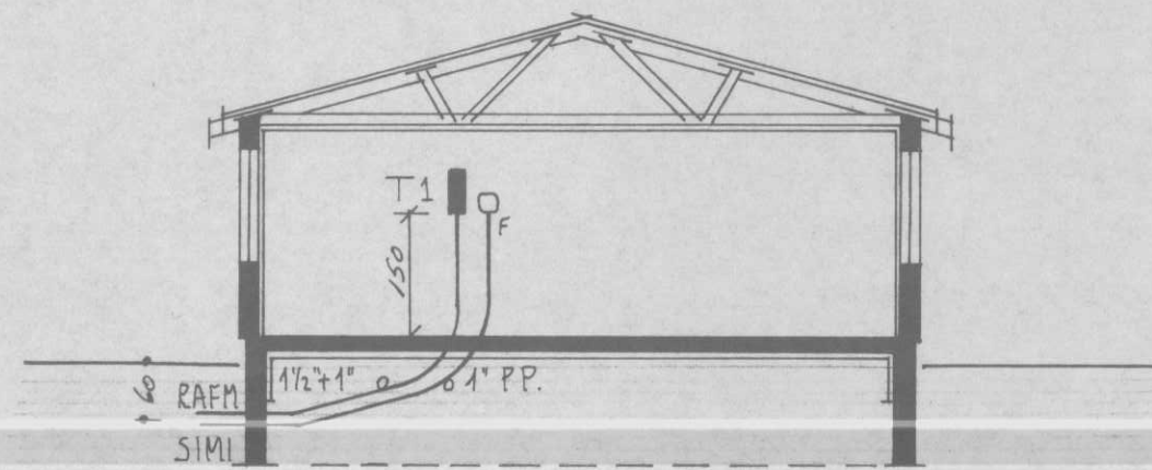
ÞVERSNEIÐING A-A.
