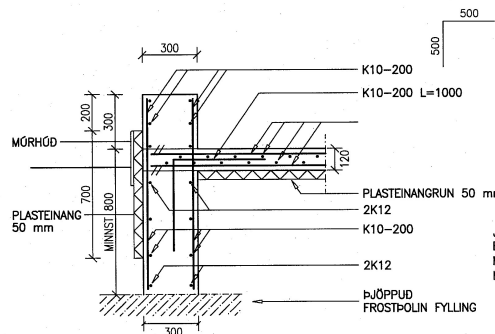
SNID 1-1 1:20
