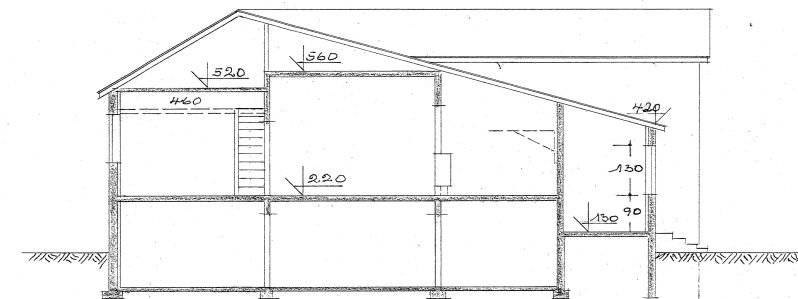
Sneiding b-b
