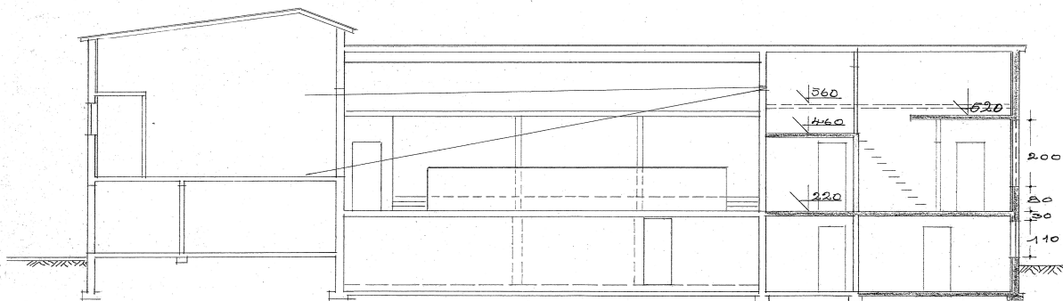
Sneiding a-a
