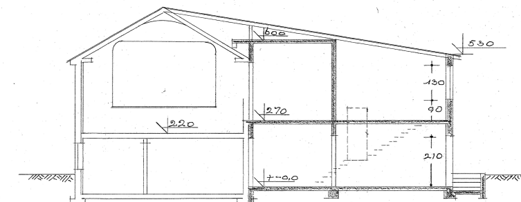
Sneiding c-c
