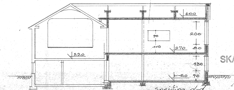
Sneiding d-d
