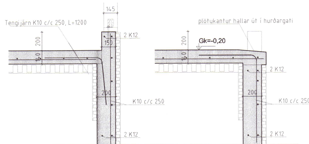
Snið U4 1:20
