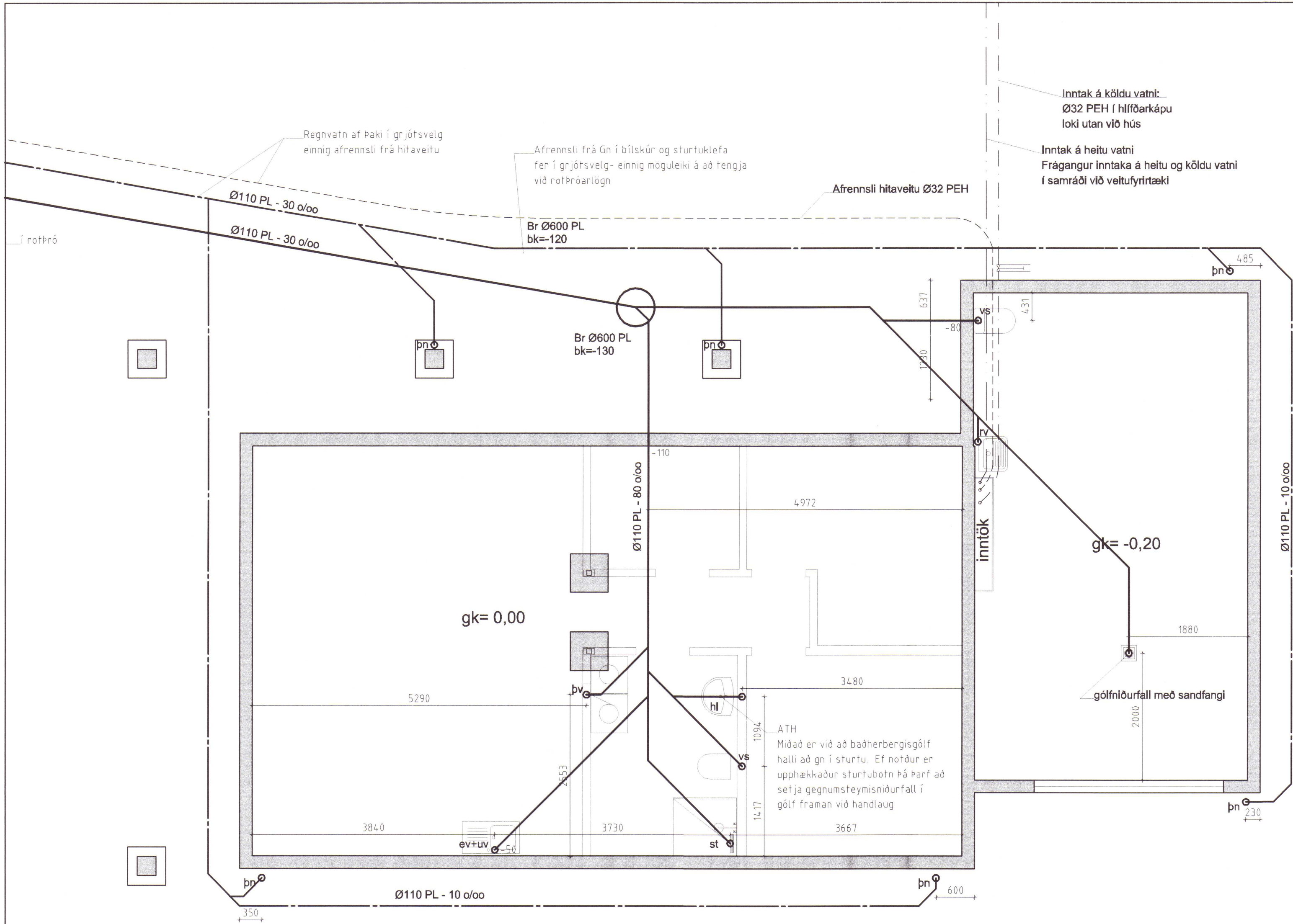
Grunnmynd 1:50
