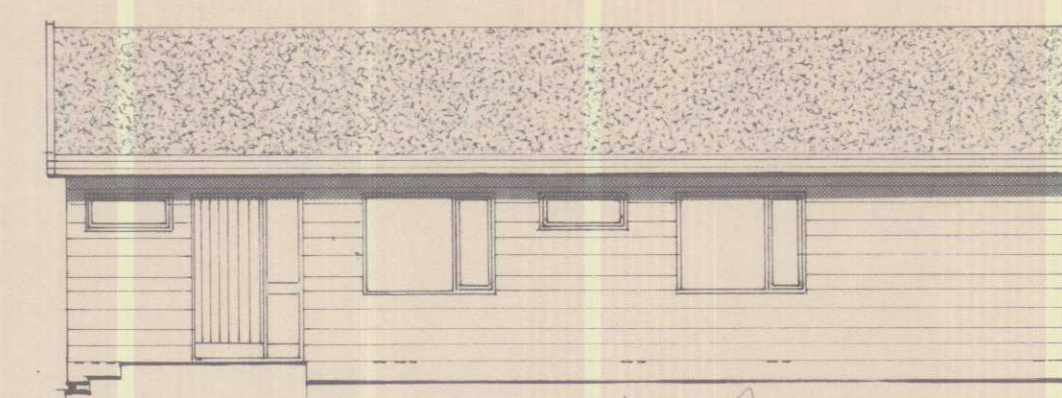
Útlitsmyndir, 1:100
