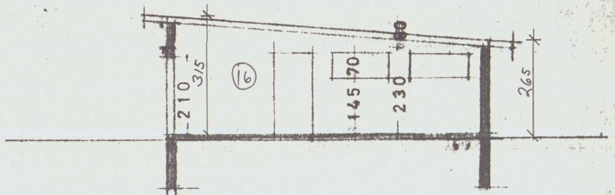
SNEIÐING A-B
