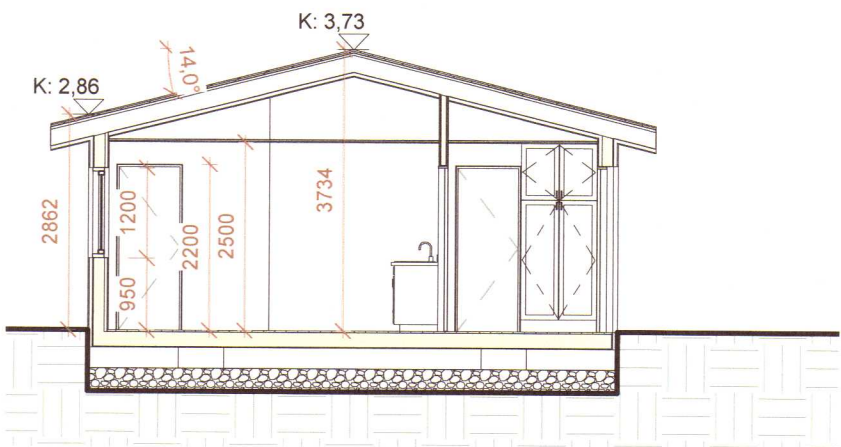
Snið A 1 : 100
