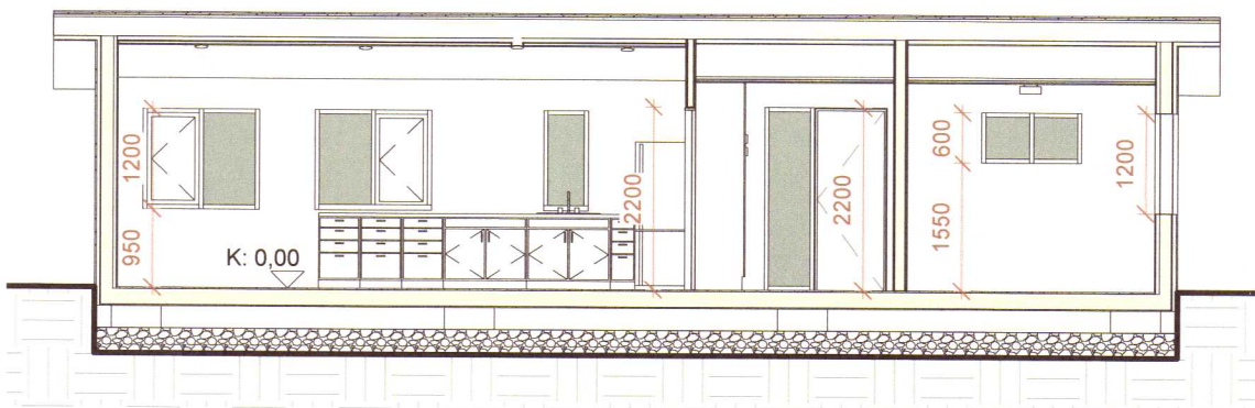
Snið B 1 : 100
