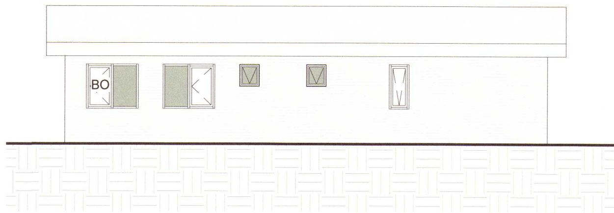
Vestur 1 : 100
