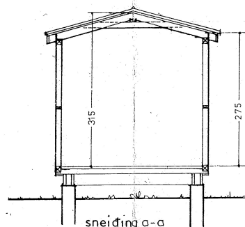
sneiding a-a
