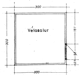
Grunnmynd mál 1:50
