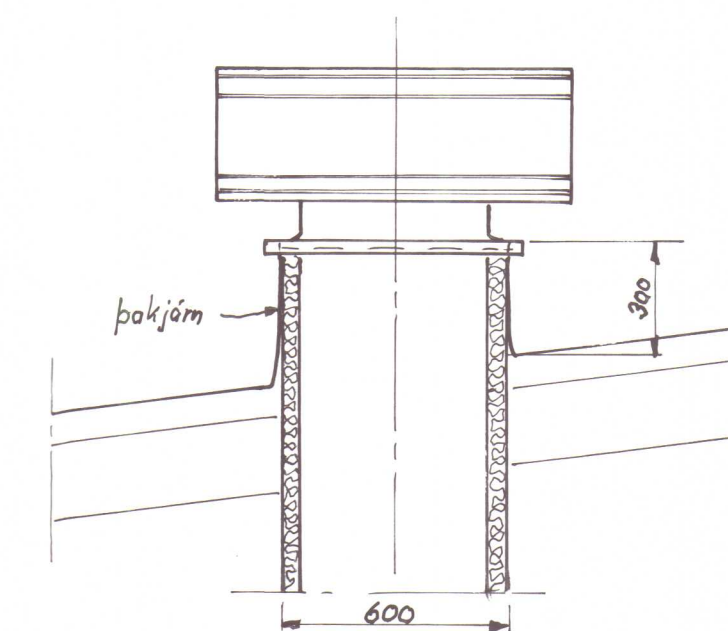
ÞAKHETTA MKV 1:20.
