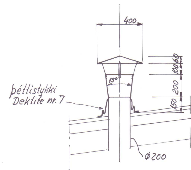
ÞAKHETTA MKV 1:20
