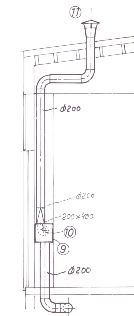
SNID B-B MKV 1:50
