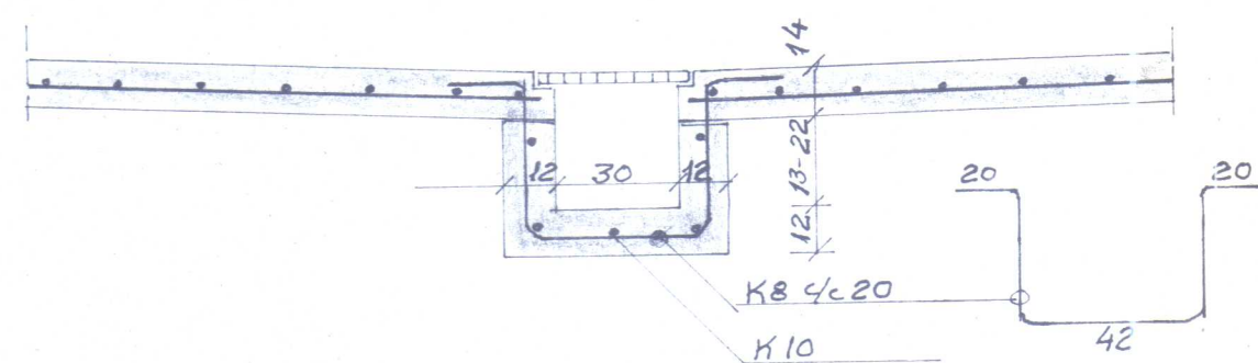
Unit A-A, , 1:20
