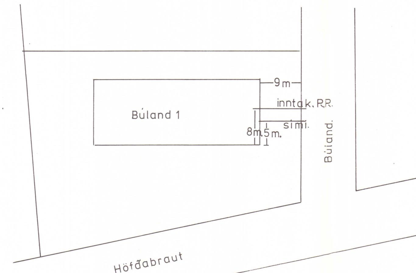
afstöðumynd 1:500
