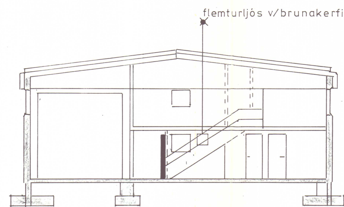
sníð 1:100 A-A
