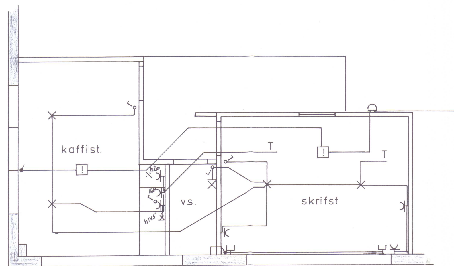
efrihæð 1:50
