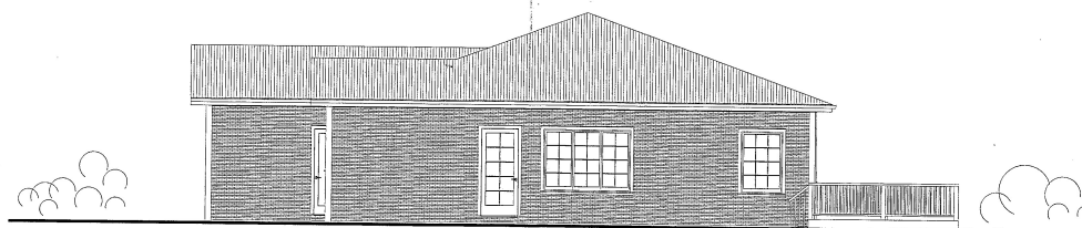
SUÐURHLÍÐ, 1:100
