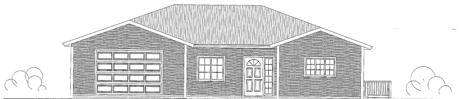
VESTURHLÍÐ, 1:100
