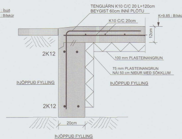
SNID D-D MKV. 1:10
