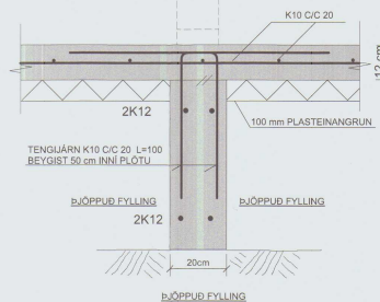
SNID E-E MKV. 1:10
