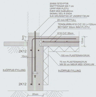
SNID E-E MKV. 1:10
