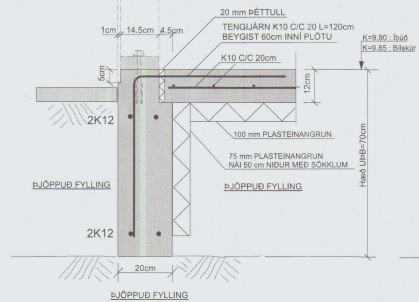
SNID C-C MKV. 1:10
