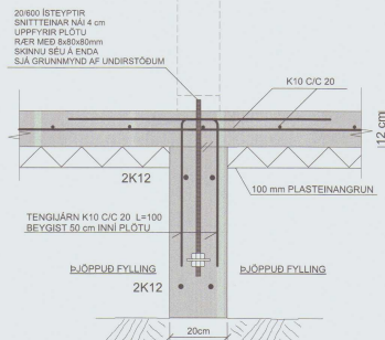
SÚLUUNDIRSTAÐA : U1, MKV. 1:10
