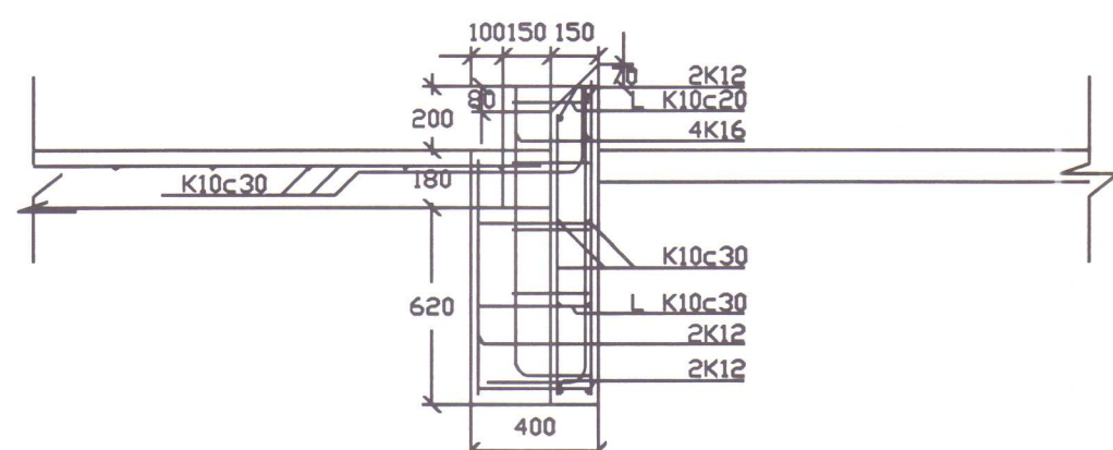
SNID B-B MKV. 1:25
