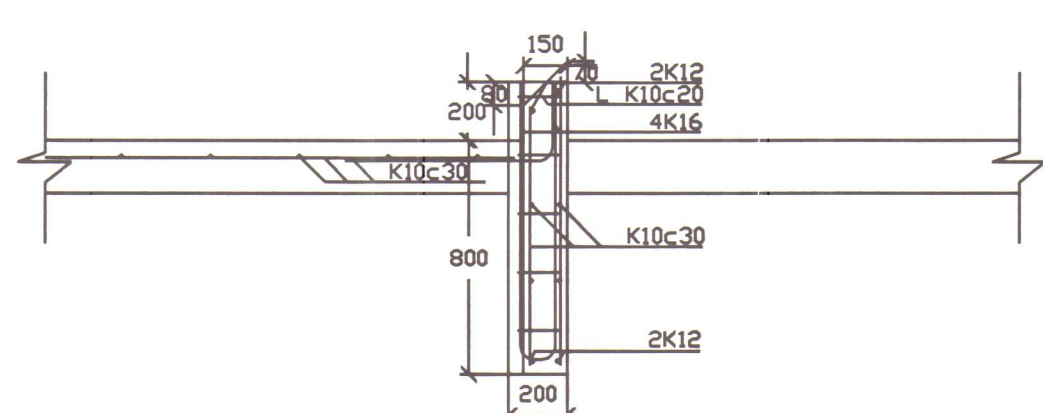
SNID A-A MKV 1:25
