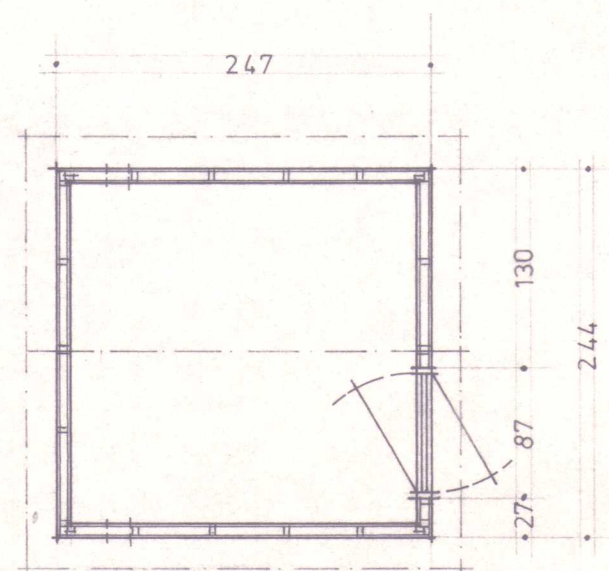
GRUNNMYND
