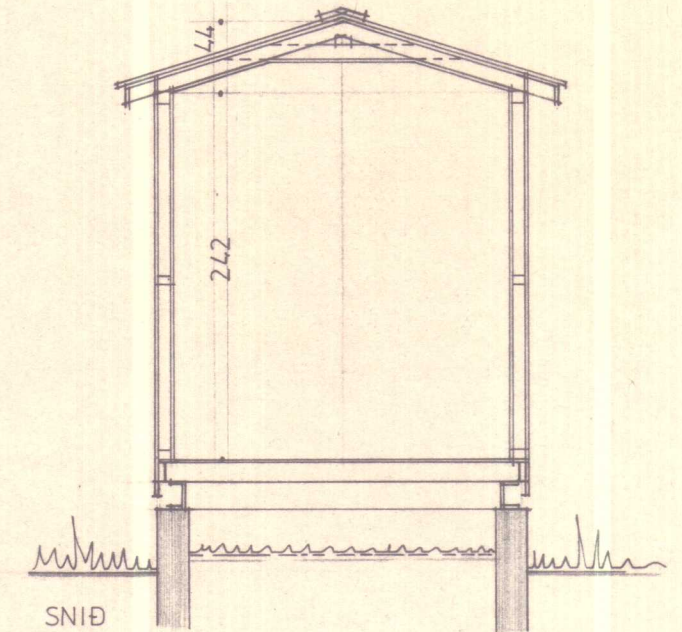
SNIÐ
