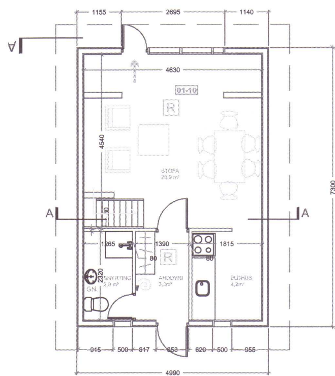
GRUNNMYND 1 HÆÐAR Í MKV. 1:100
