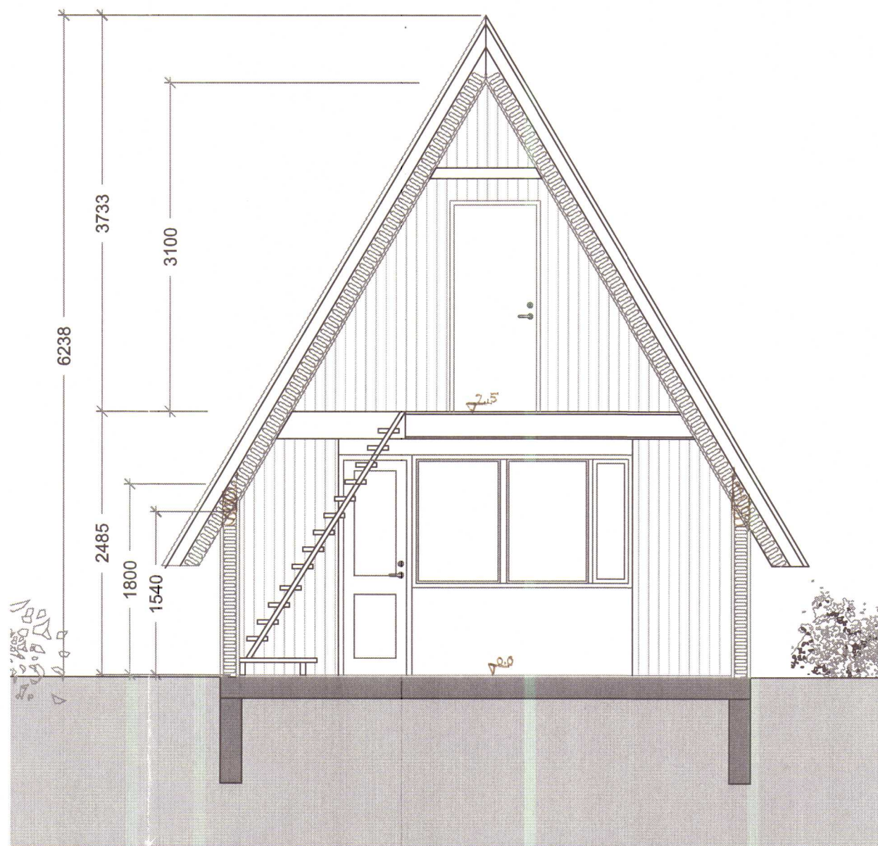
SNEIÐMYND A-A Í MKV. 1:50
