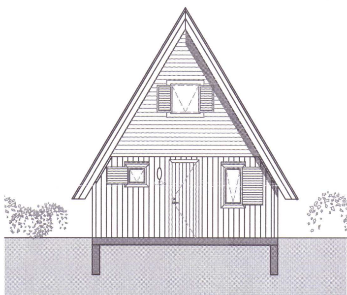
ÚTLIT FRAMHÚÐ Í MKV. 1:100
