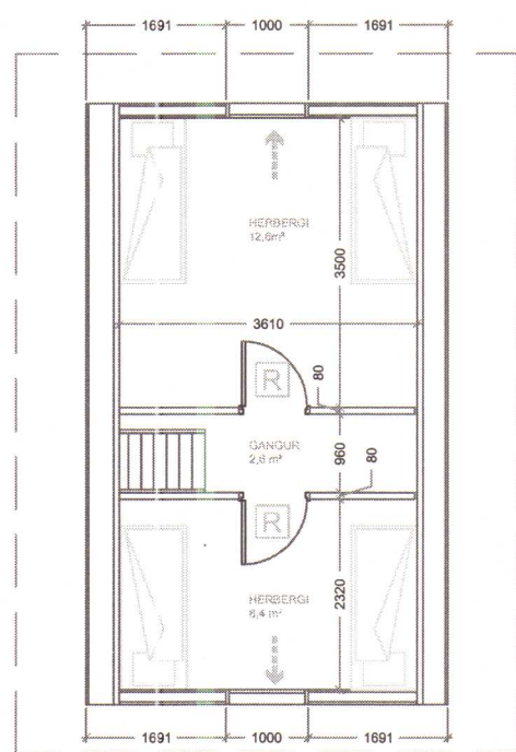
GRUNNMYND 2 HÆÐAR Í MKV. 1:100
