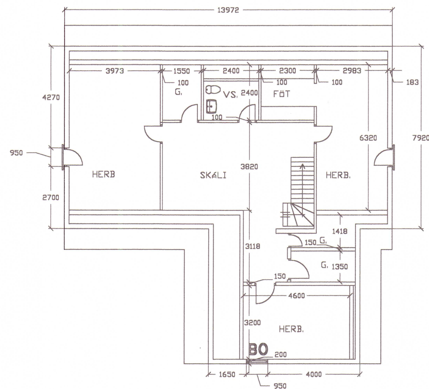
RISHÆÐ 1:100
