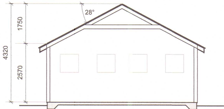
SNÍÐ A mkv. 1:100
