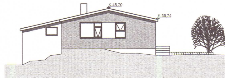
útlit Suður
