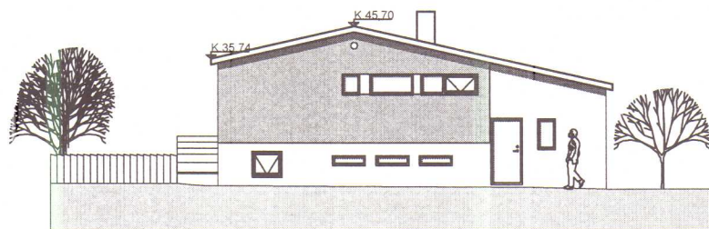
útlit Norður
