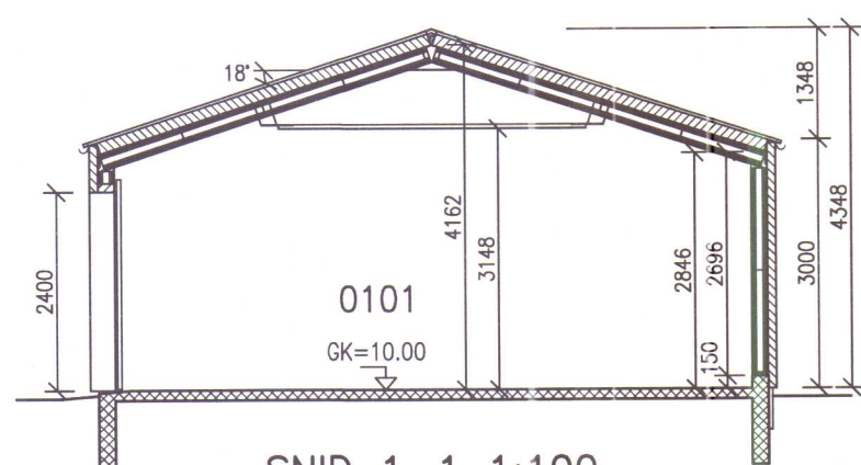
SNID 1-1 1:100
