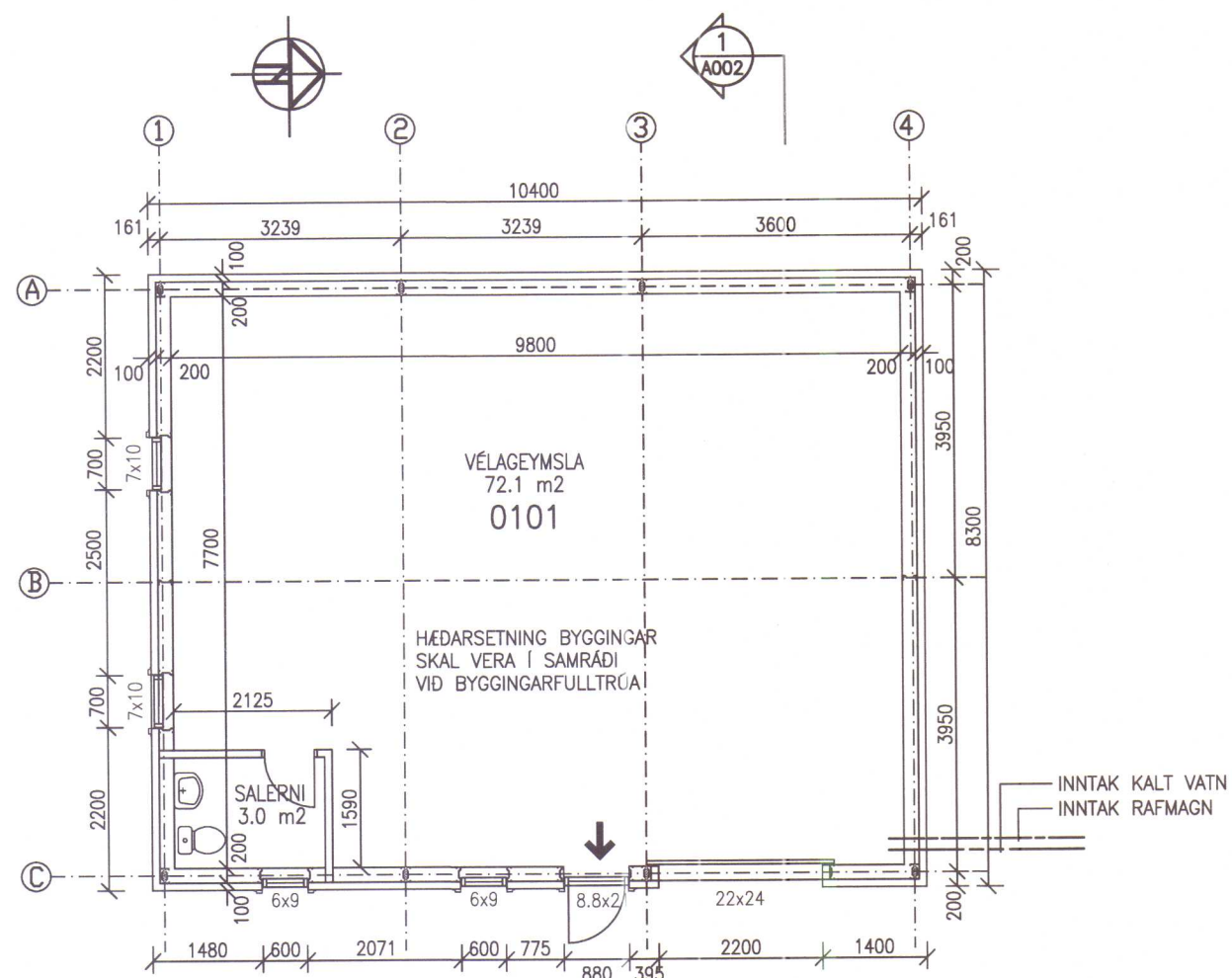
GRUNNMYND 1:100
