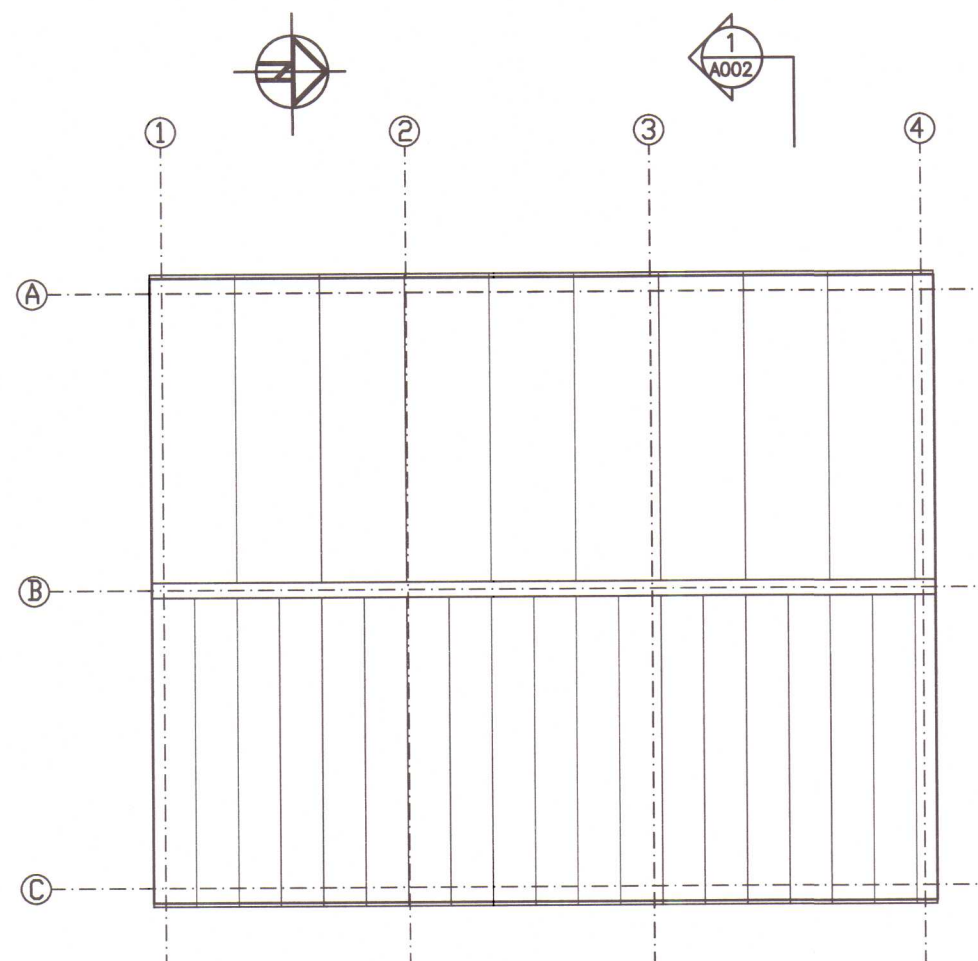
ÚTLIT VESTURHLIÐ
