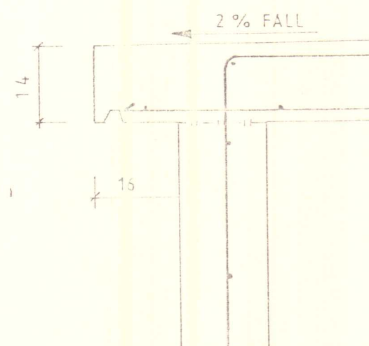
ÞAKBRÚN M=1:10
