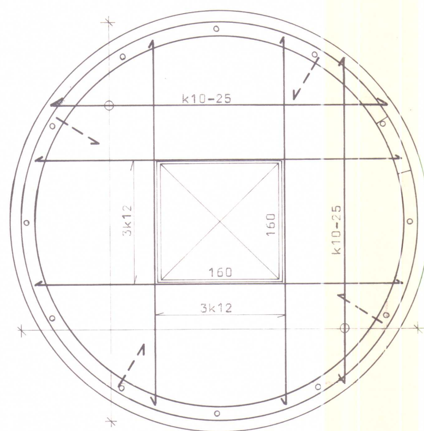
ÞAKPLATA, M=1:50
