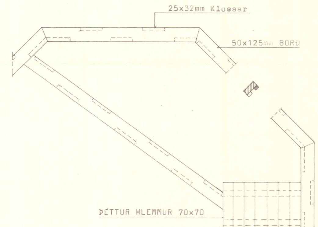
FRÁRENNSLI Á GÓLFÍ Í VOTHEYSTURNI M=1:20
