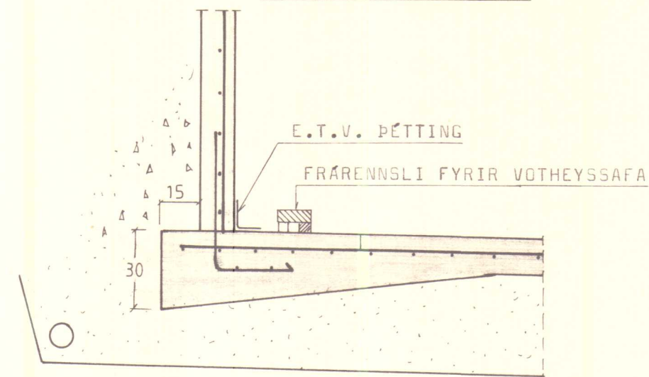
I M=1:20
