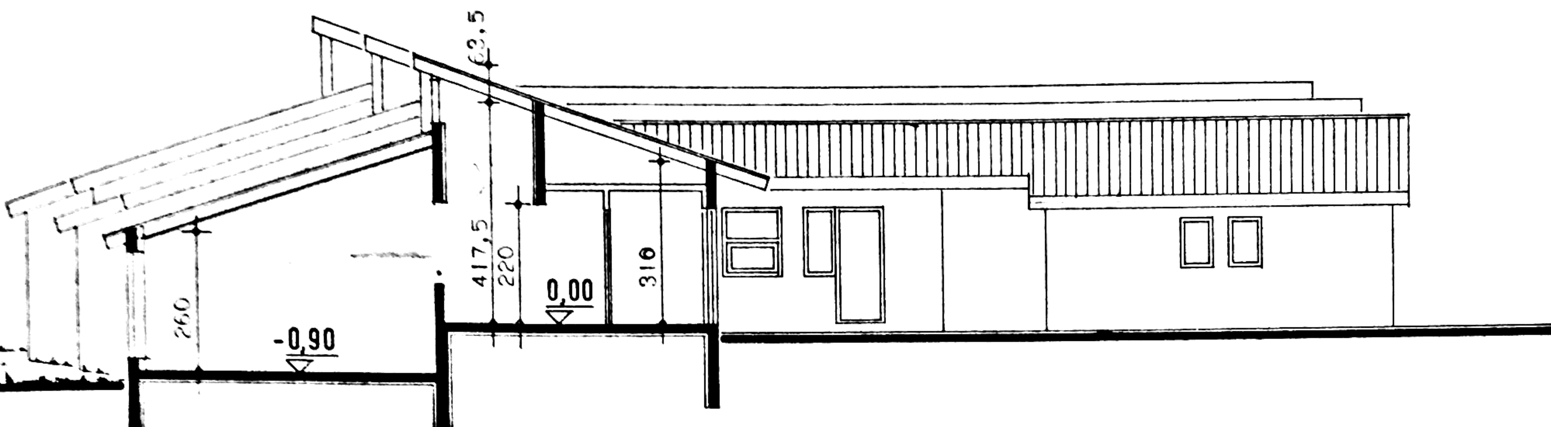
SNEIÐING A-A
