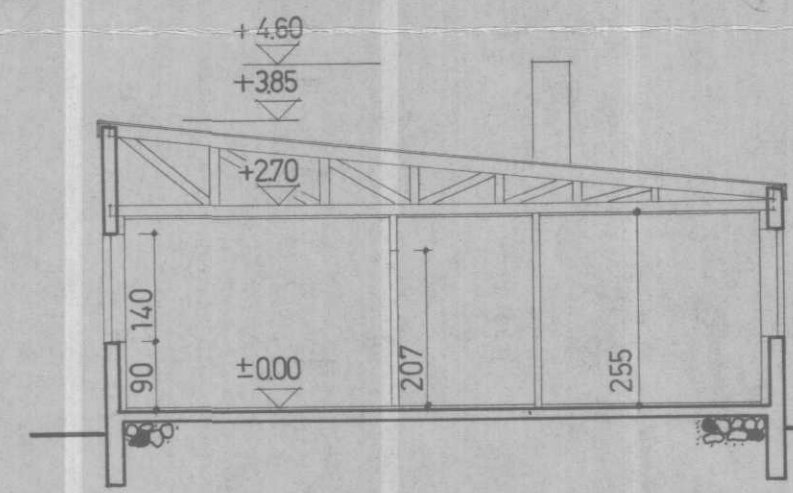
SKURÐUR A-A M. 1:100
