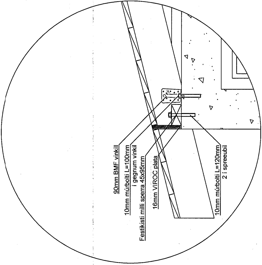
DEILI A, MKV. 1:10
