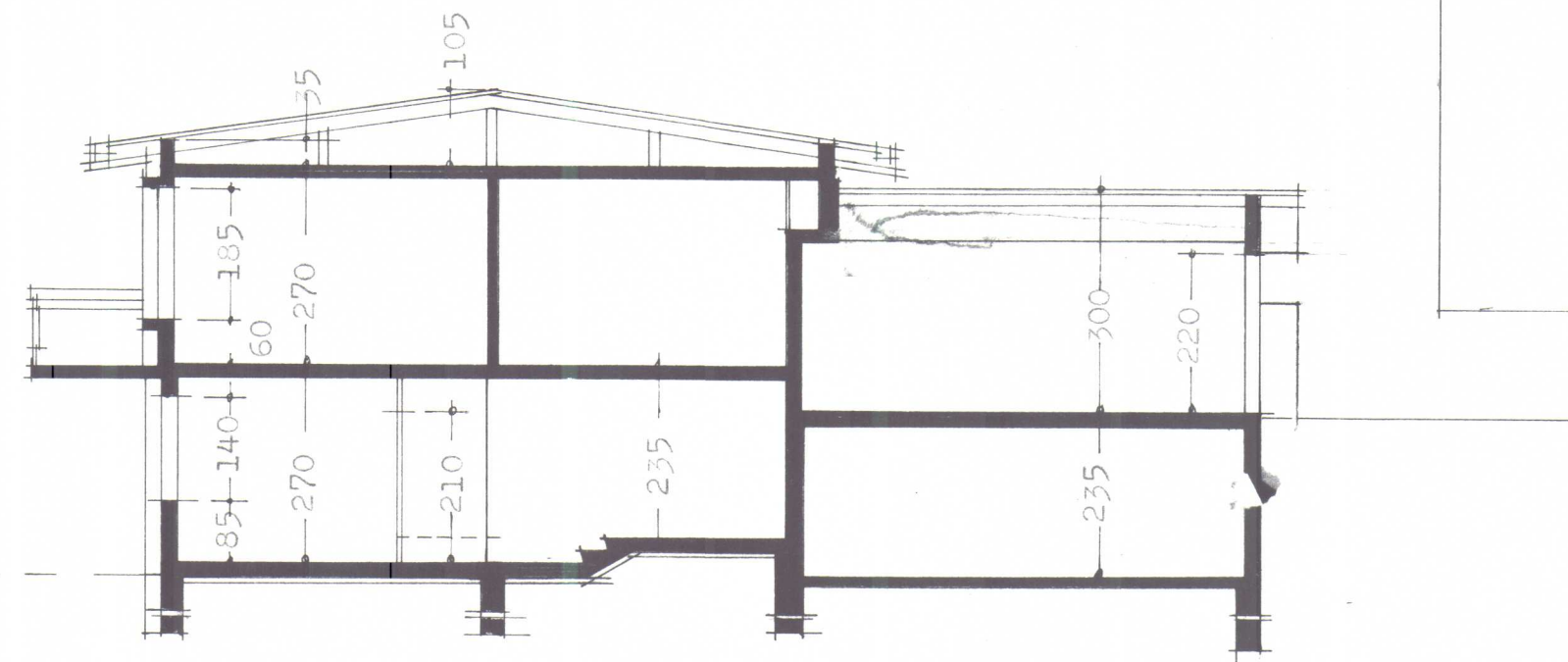
skurður A-A
