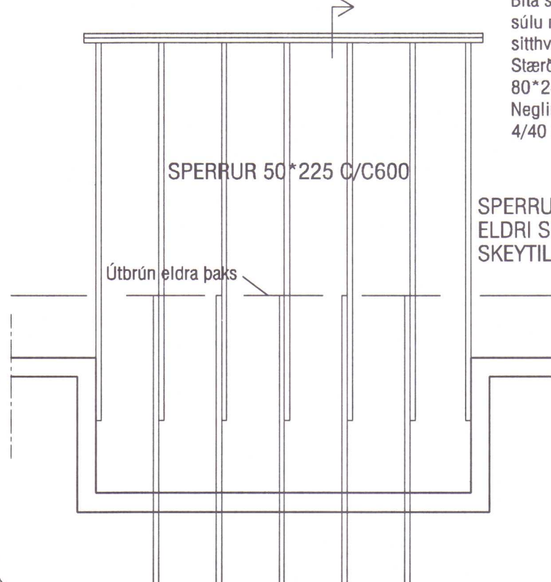
GRUNNMYND ÞAKS
