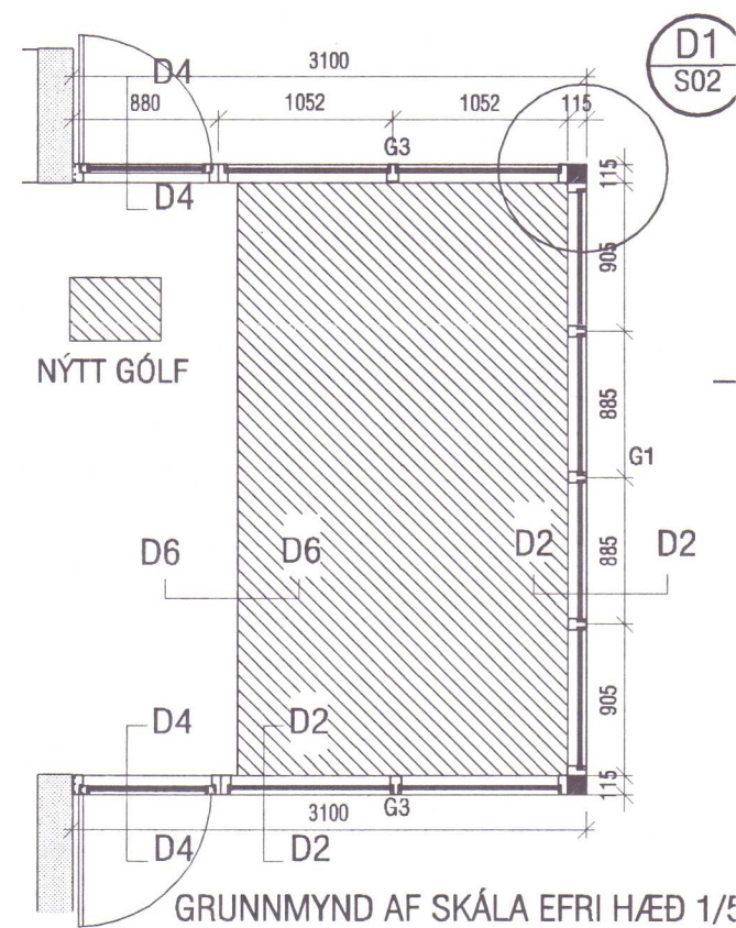
GRUNNMYND AF SKÁLA EFRI HÆÐ 1/50
