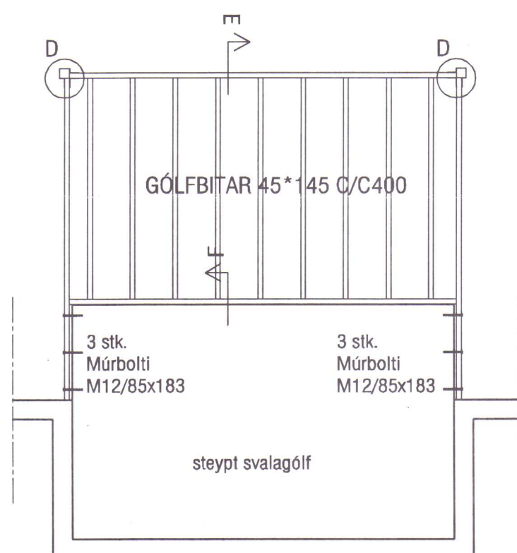
GRUNNMYND MILLIGÓLF
