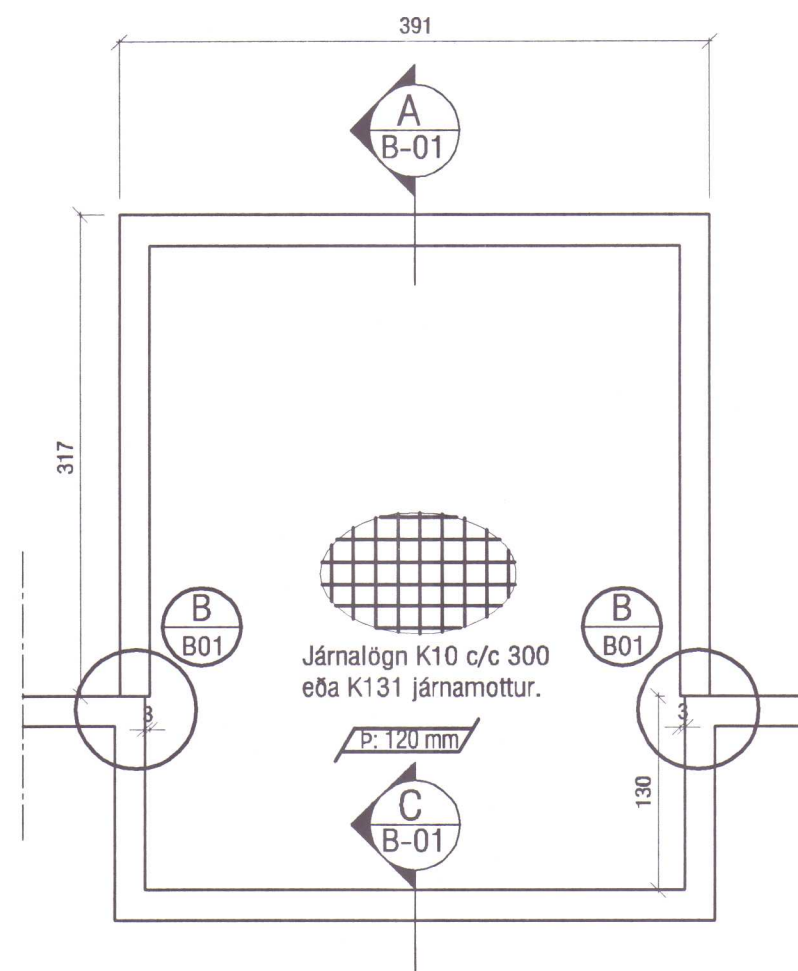
GRUNNMYND MILLIGÓLF
