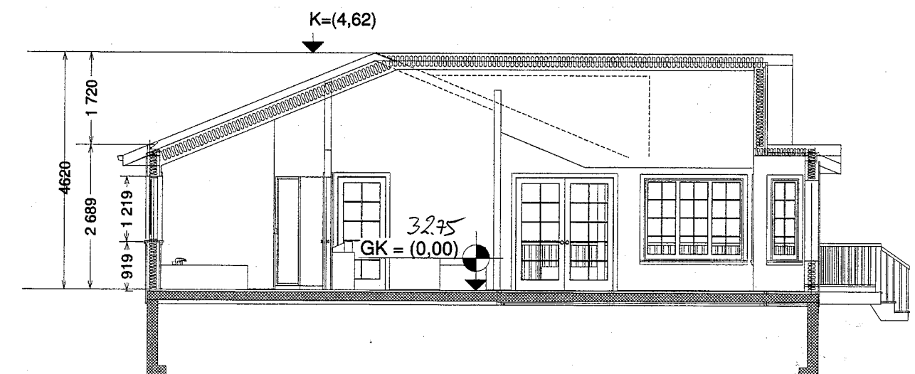
SKURÐUR A, 1:100
