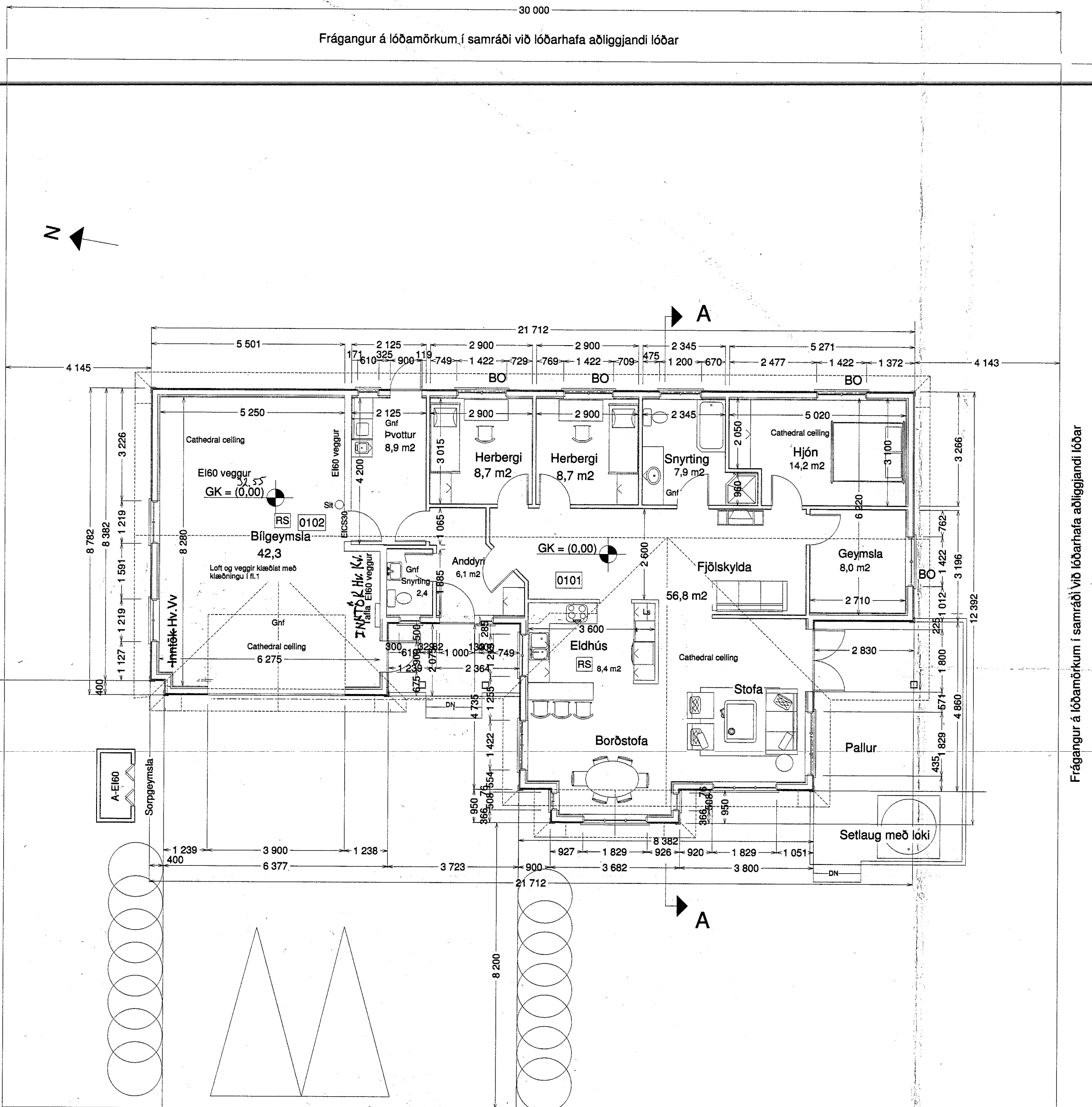
GRUNNMYND, 1:100
