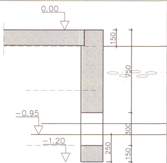
KÓTAR, SKÝRINGAR Mkv. 1:20
