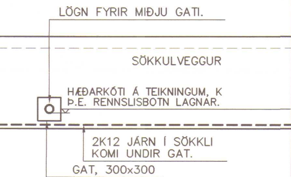
KÓTAR, SKÝRINGAR Mkv. 1:50
