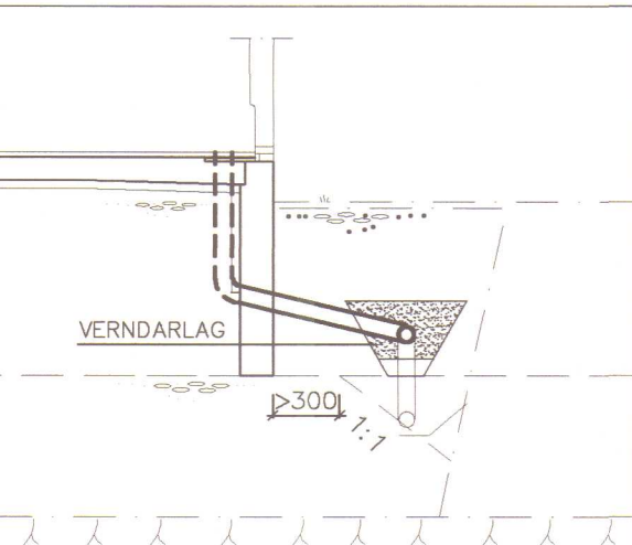
SNID VIÐ SÖKKUL Mkv. 1:50
