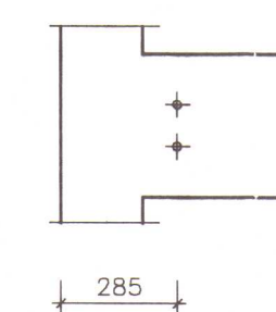
FESTIBOLTAR ø20 Í ÁS 1 OG 6 (BOLTAR SJÁ LÍNU A)
