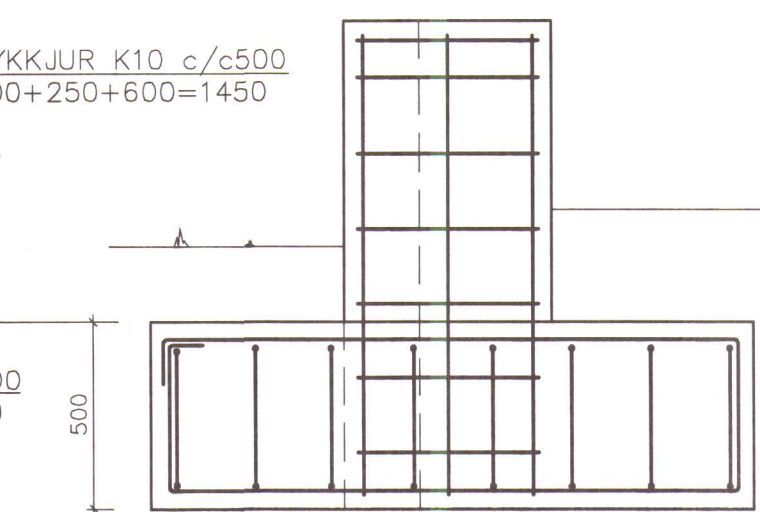
SÚLUR A, 2-5
