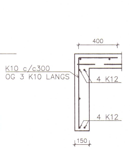
SNID D-D
