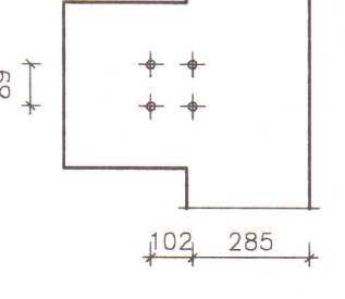
YFIRBORD STEYPU
