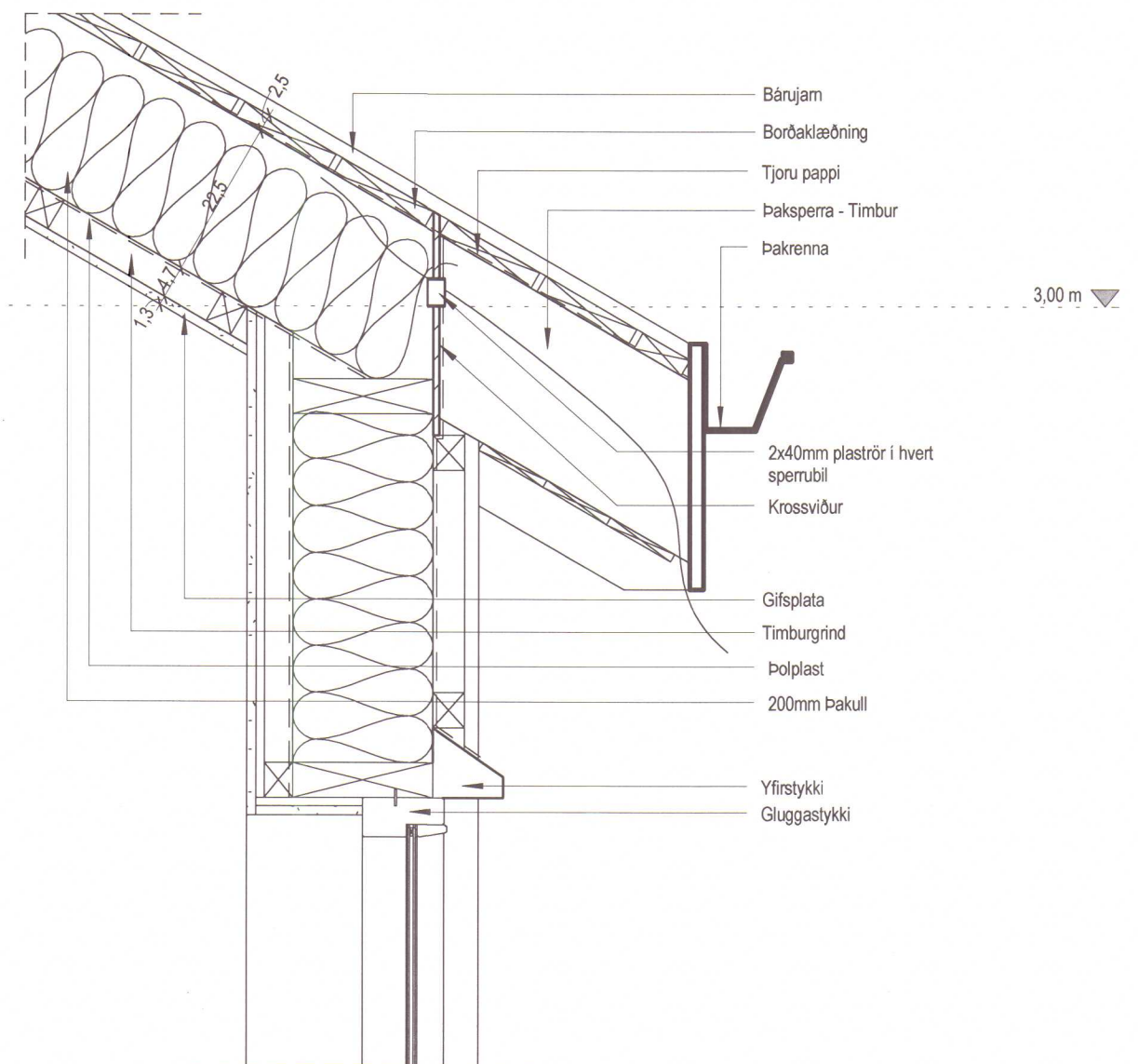
Deili 02 1 : 10
