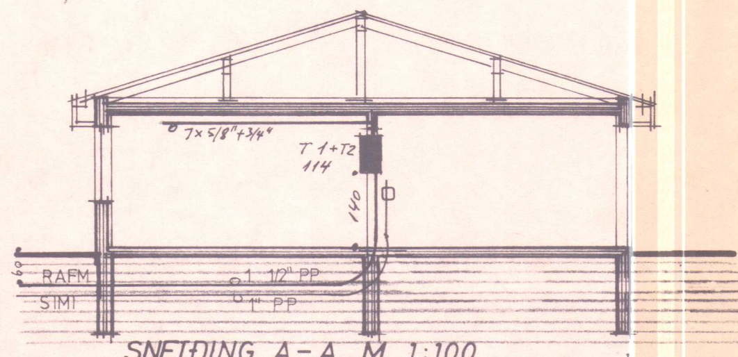
SNEDING A-A M 1:100
