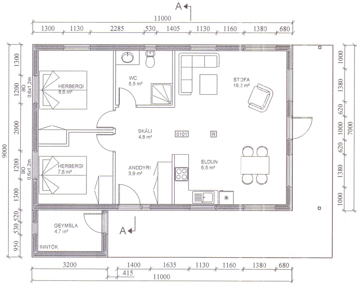
GRUNNMYND Mkv. 1:100
