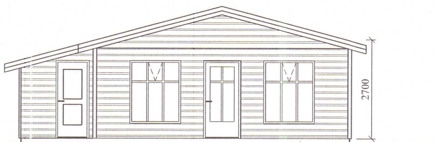
SUÐURHLID Mkv. 1:100
