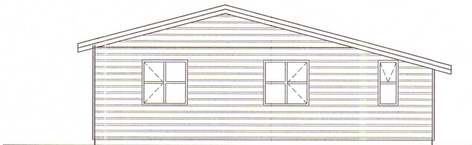
NORÐURHLID Mkv. 1:100
