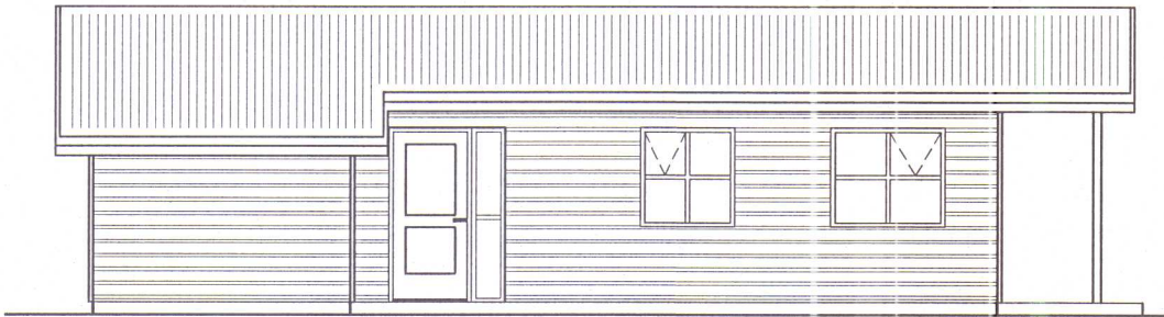
VESTURHLID Mkv. 1:100
