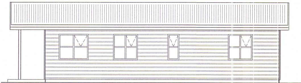
AUSTURHLID Mkv. 1:100
