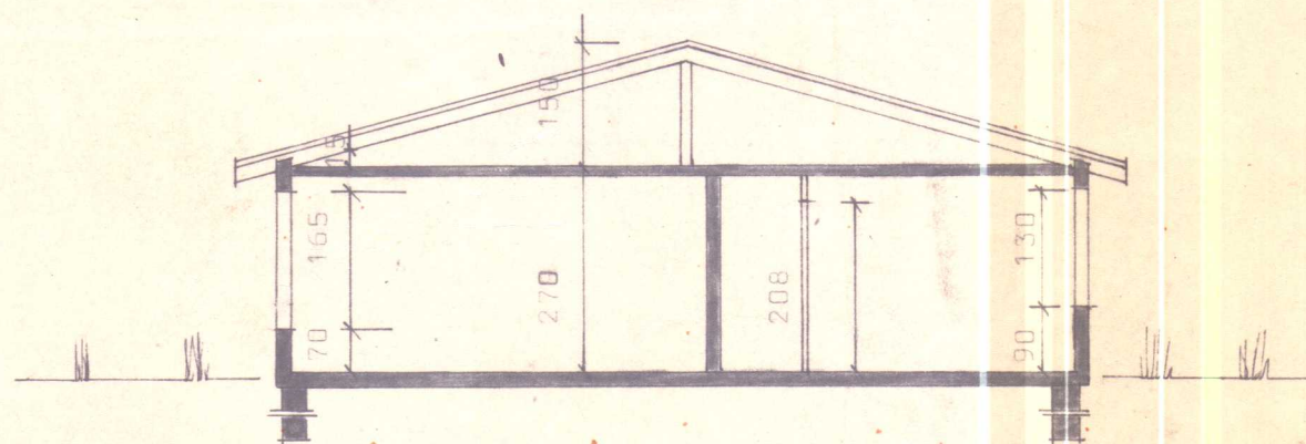
Skurður A-A.
