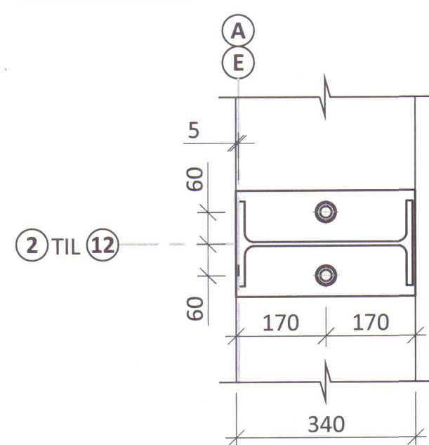
SNID X - X M1:10
