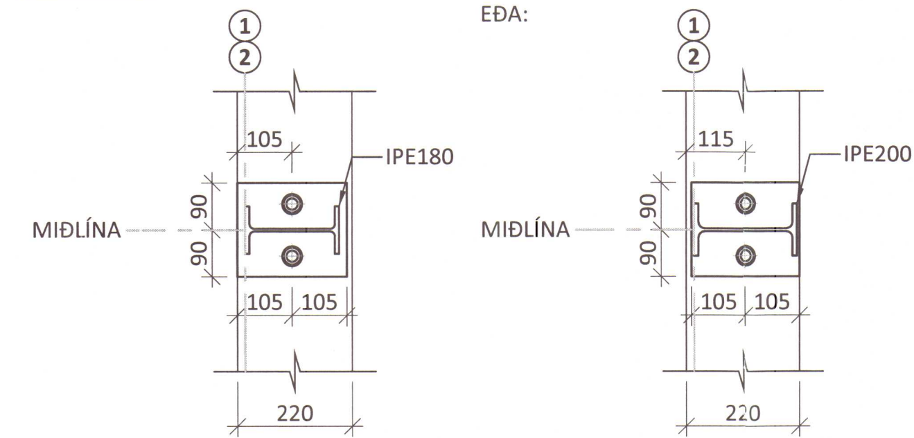
SNID Y - Y M1:10
