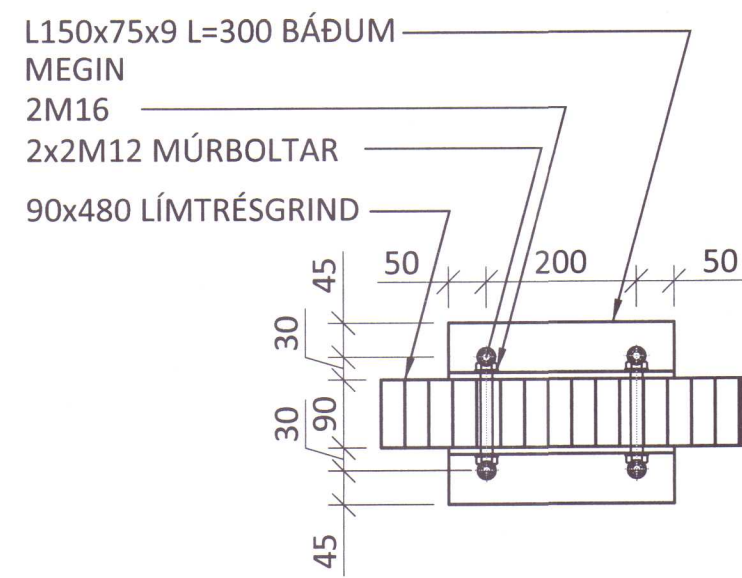
SNID Z - Z M1:10
