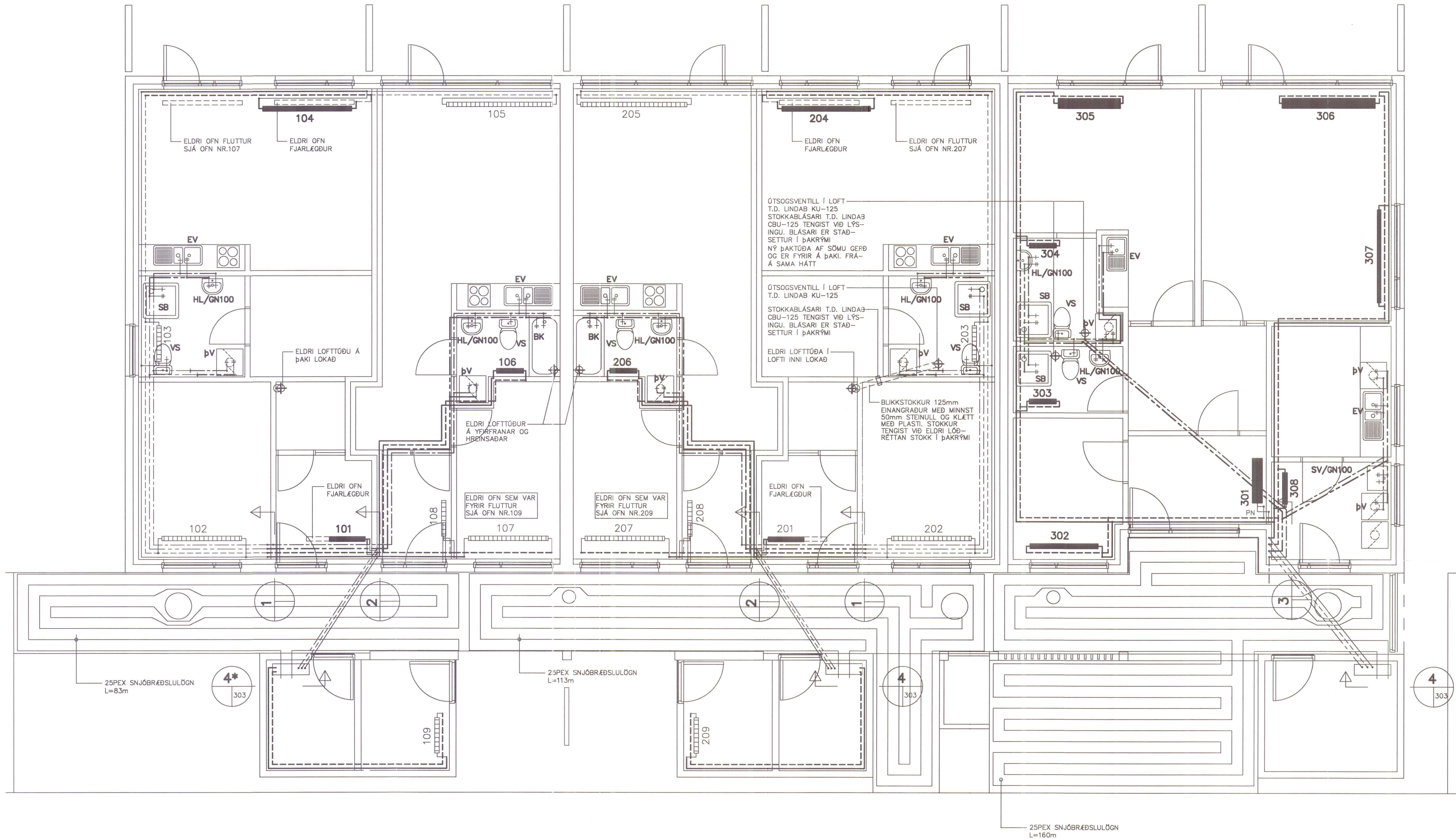
OFNASKRÁ FYRIR HÚS NR.10: AFKÖST OFNA MIÐUÐ VÍÐ ΔT=35°C
