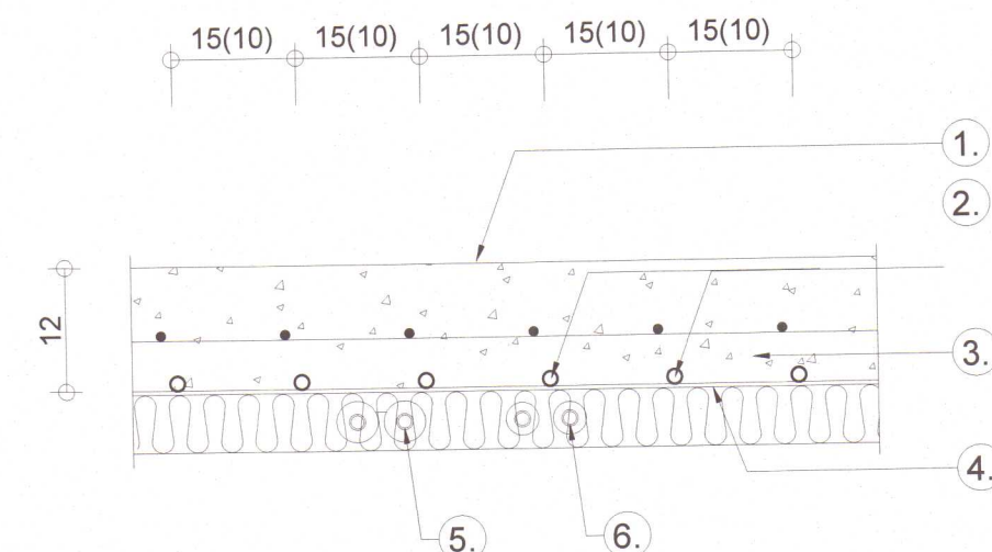
SNİÐ Í BOTNPLÖTU mkv. 1:10
