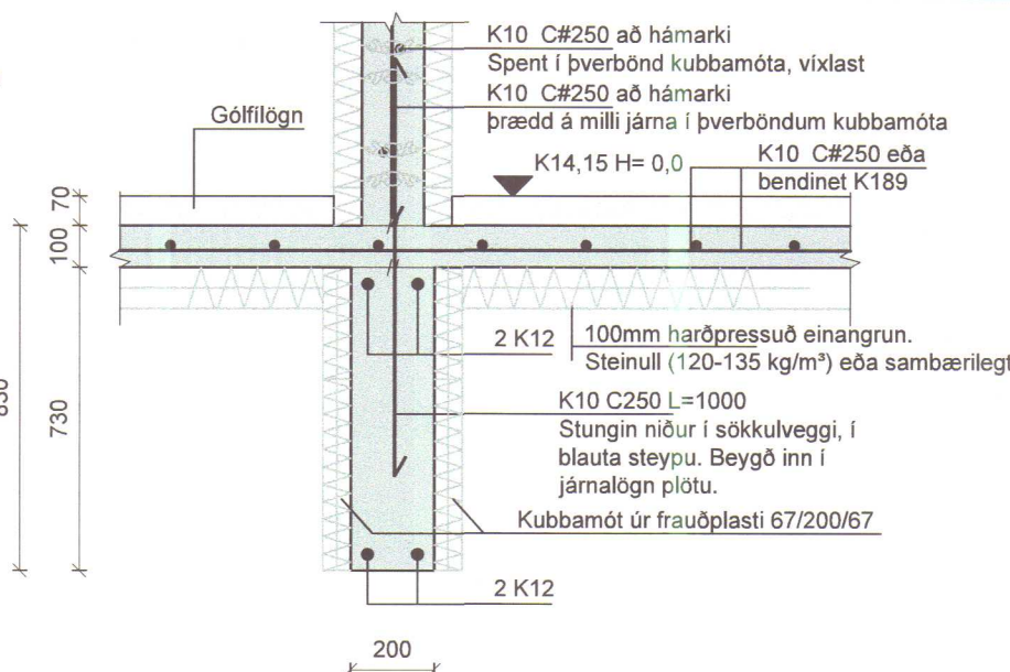
Snið J mkv. 1:20
