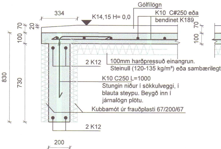
Snið H mkv. 1:20
