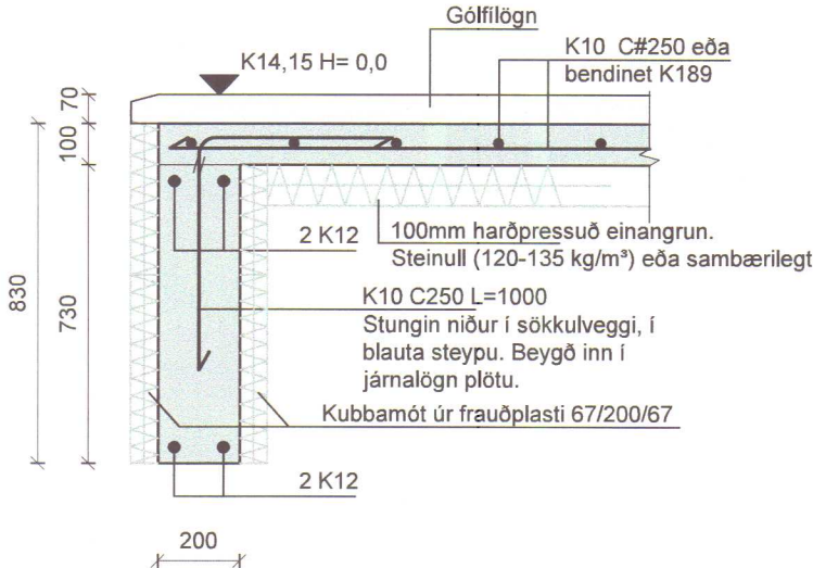
Snið G mkv. 1:20
