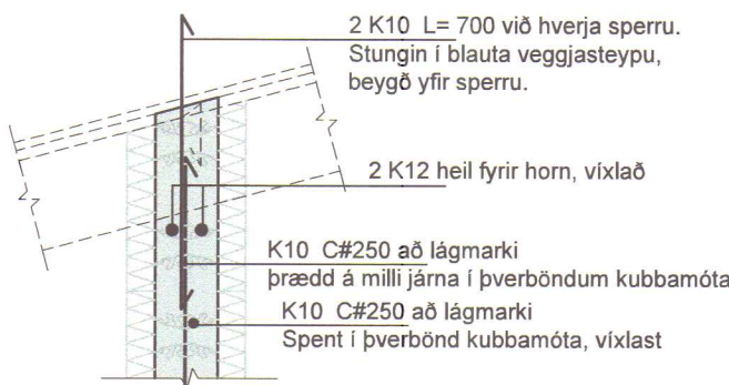
Snið G mkv. 1:20
