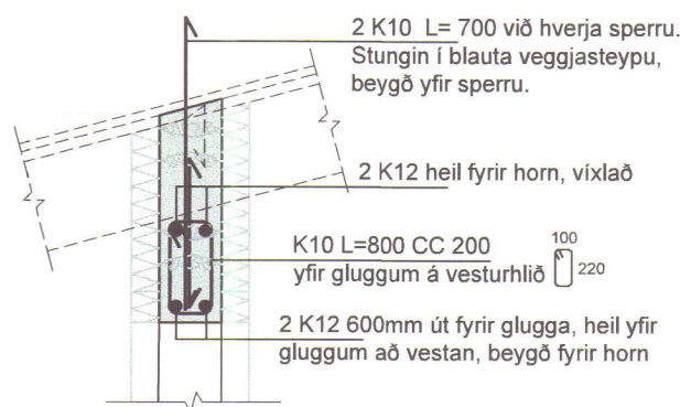
Snið H mkv. 1:20
