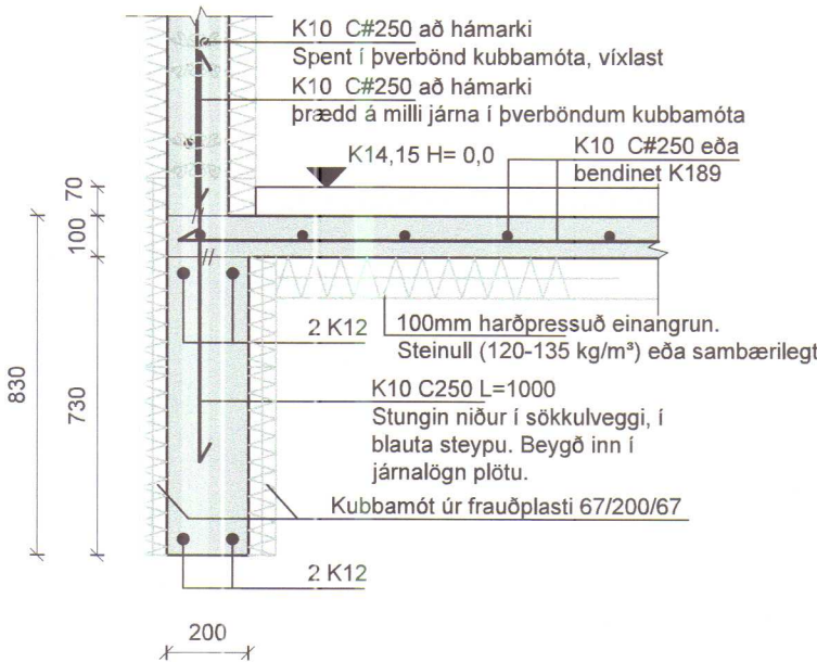
Snið F mkv. 1:20
