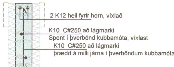
Snið J mkv. 1:20
