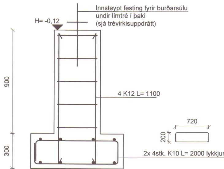
Undirstaða S1 mkv. 1:20
