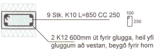
Deili 2 mkv. 1:20
