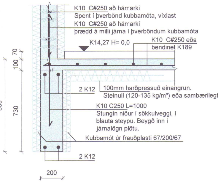
Snið F mkv. 1:20
