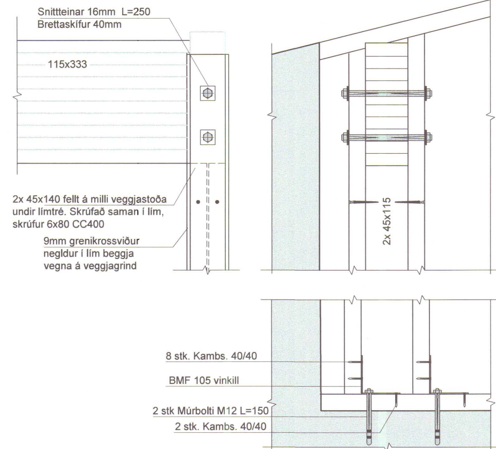
SNÍÐ T mkv. 1:10
