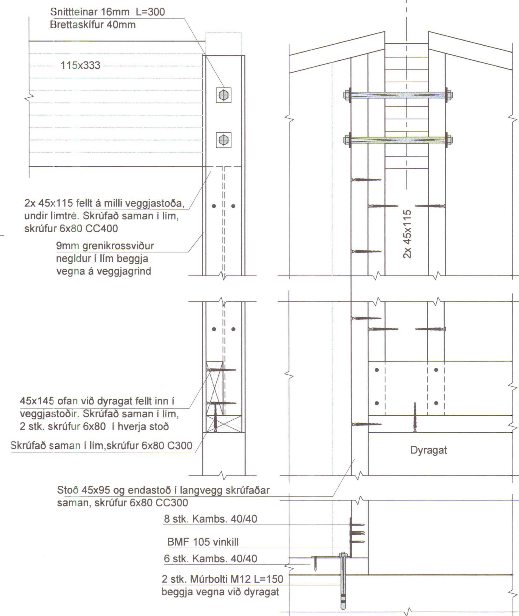
SNÍÐ R mkv. 1:10
