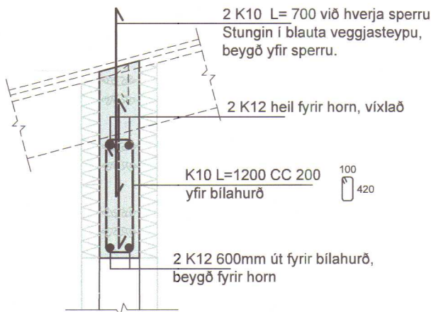
Deili 1 mkv. 1:20
