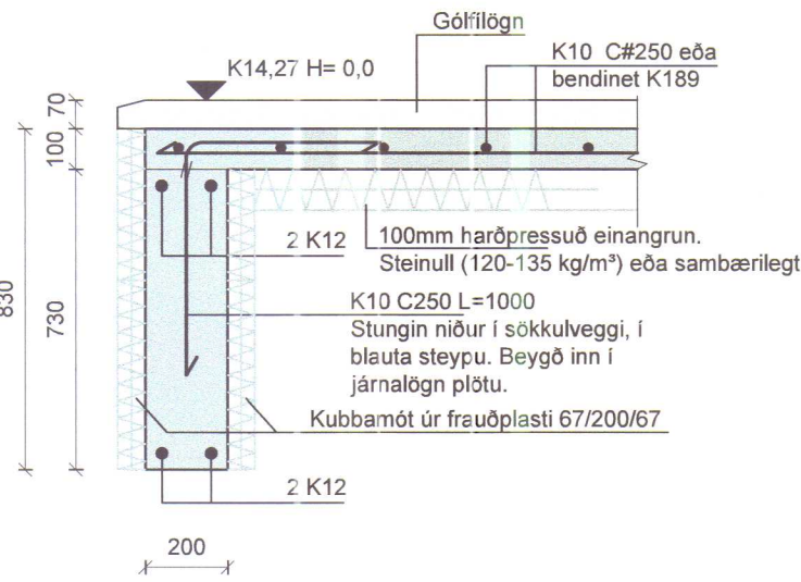
Snið G mkv. 1:20
