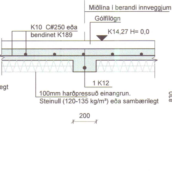
Snið I mkv. 1:20
