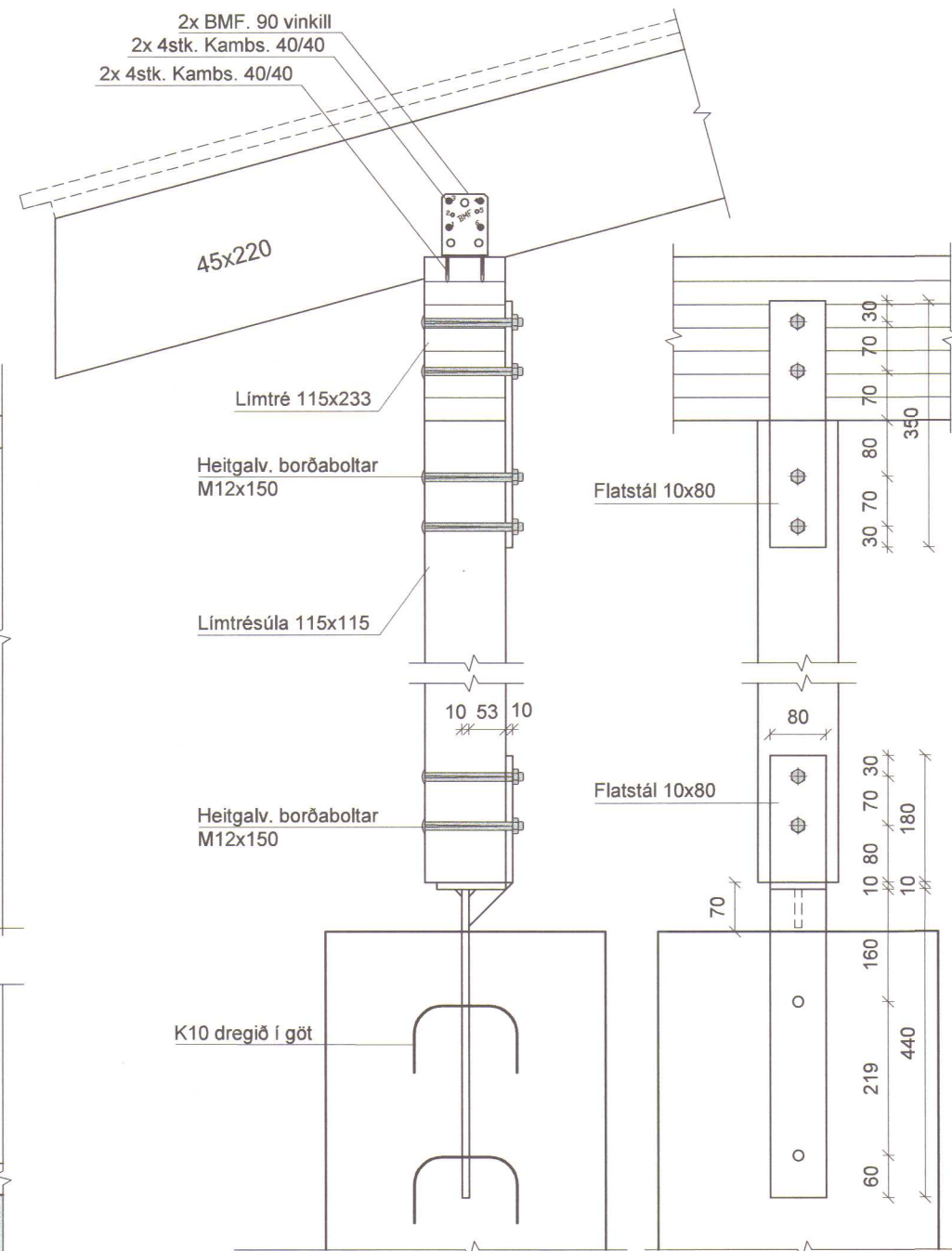
SNÍÐ U mkv. 1:10
