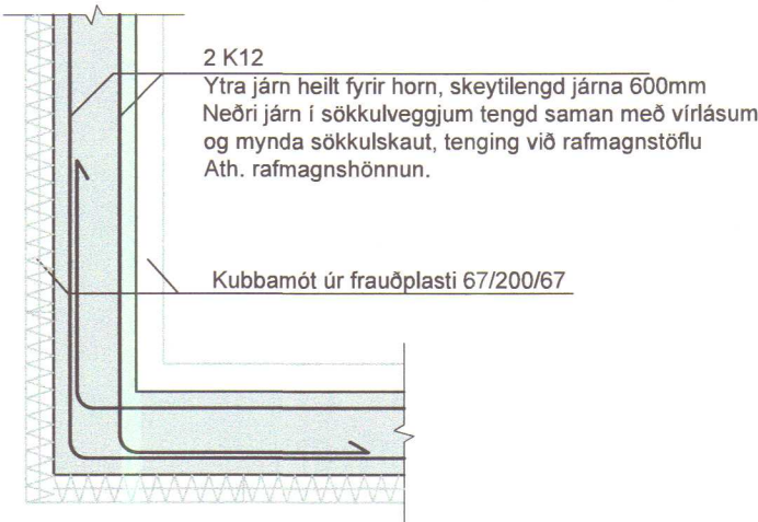
Deili 1 mkv. 1:20
