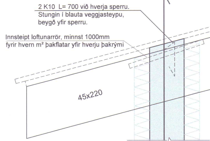
SNÍÐ P mkv. 1:10
