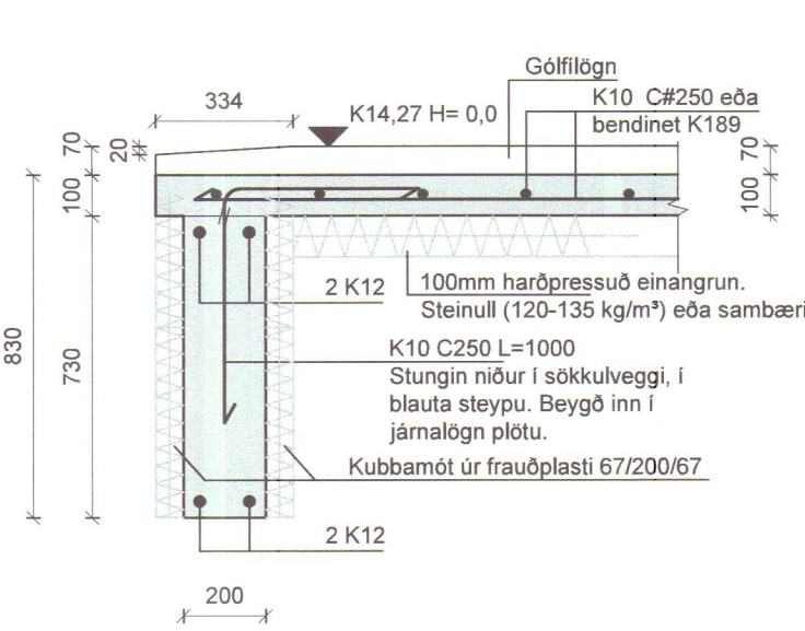
Snið H mkv. 1:20
