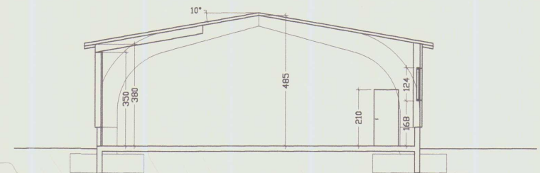
SNID A-A
