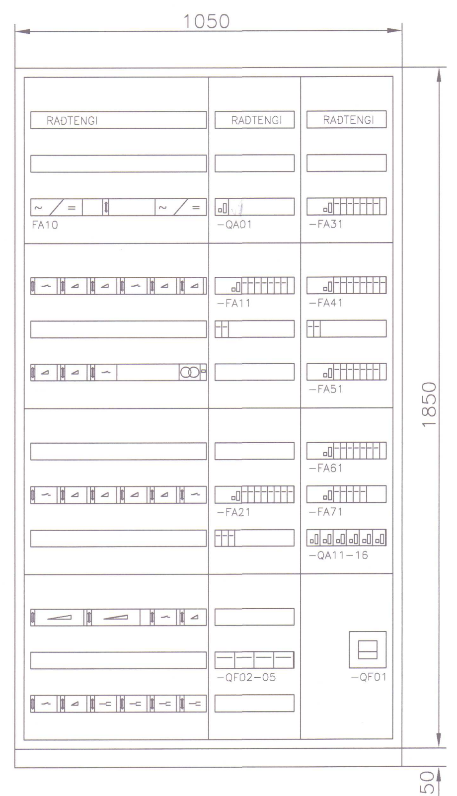
TAFLA -A11 1050x1850x275 mm Niðurröðun - Tillaga
