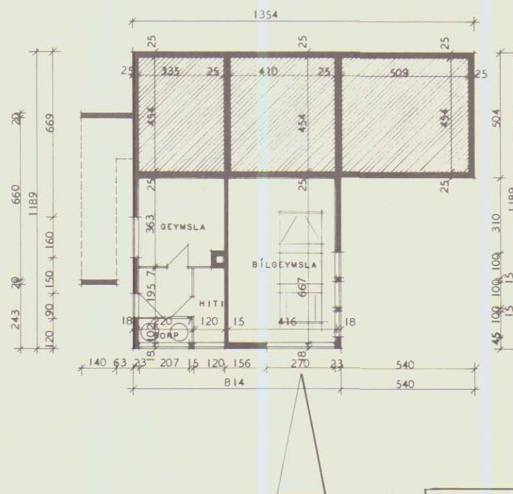
GRUNNMYND KJALLARA
