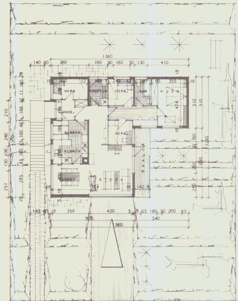
GRUNNMYND HEDAR
