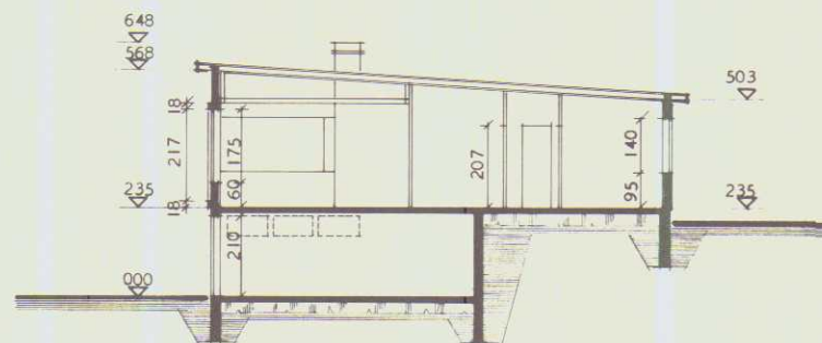
SNEIÐING
