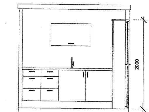
Sníð : C-C Mál. 1:50
