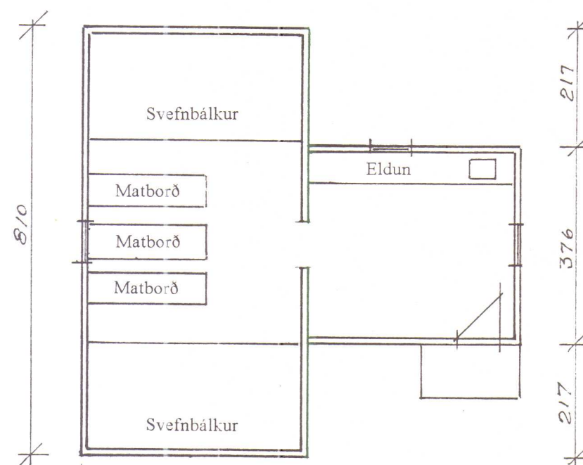
Grunnmynd
