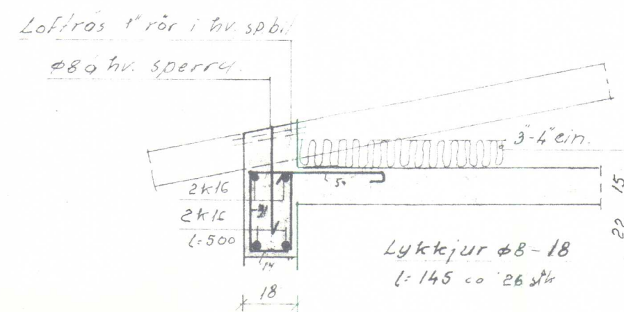
snid B. M=1:20
