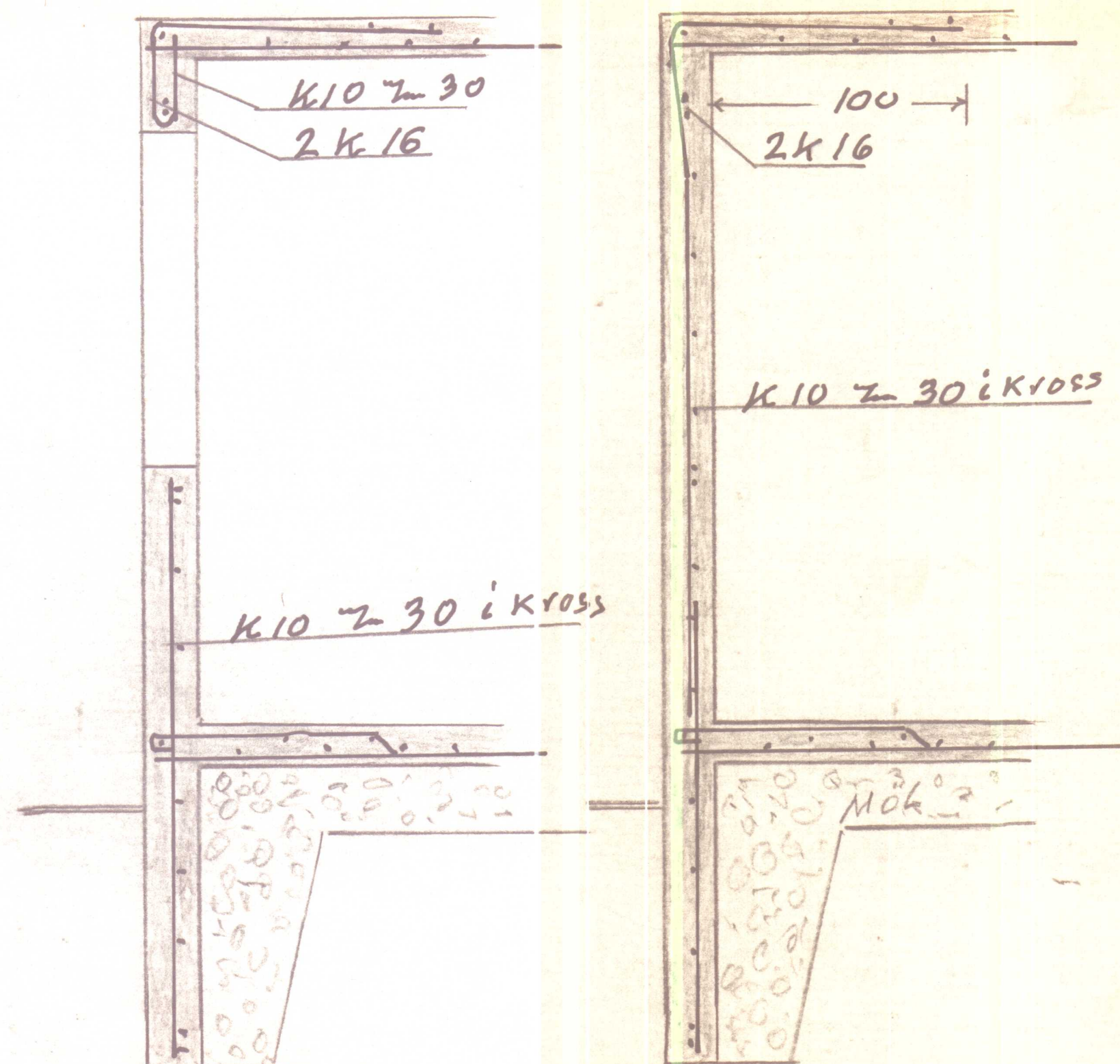
Sníð í vegg 1:20
