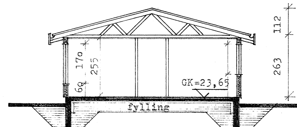
SNEIÐING A-A
