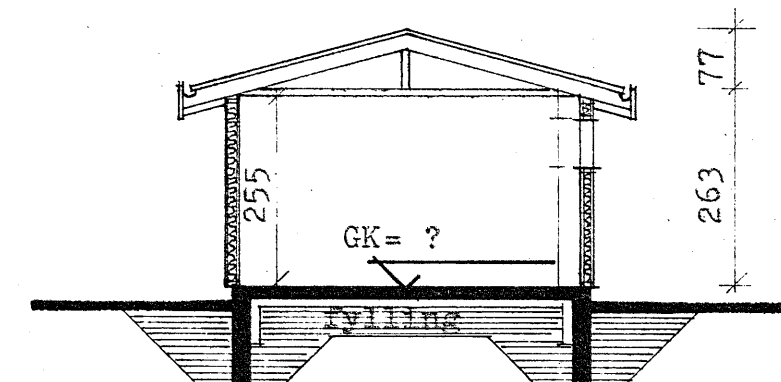
SNEIÐING B-B
