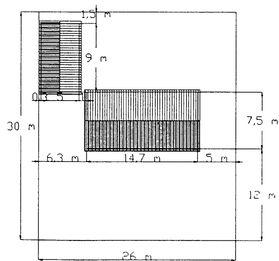
AFSTÖÐUMYND MKV. 1:500
