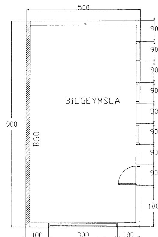
GRUNNMYND
