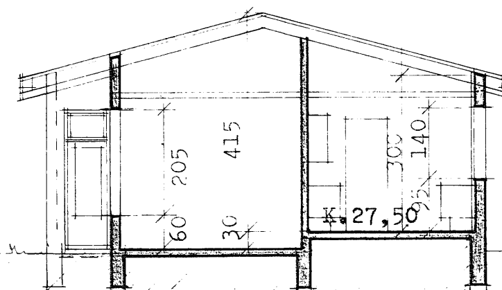
Skurður A-A
